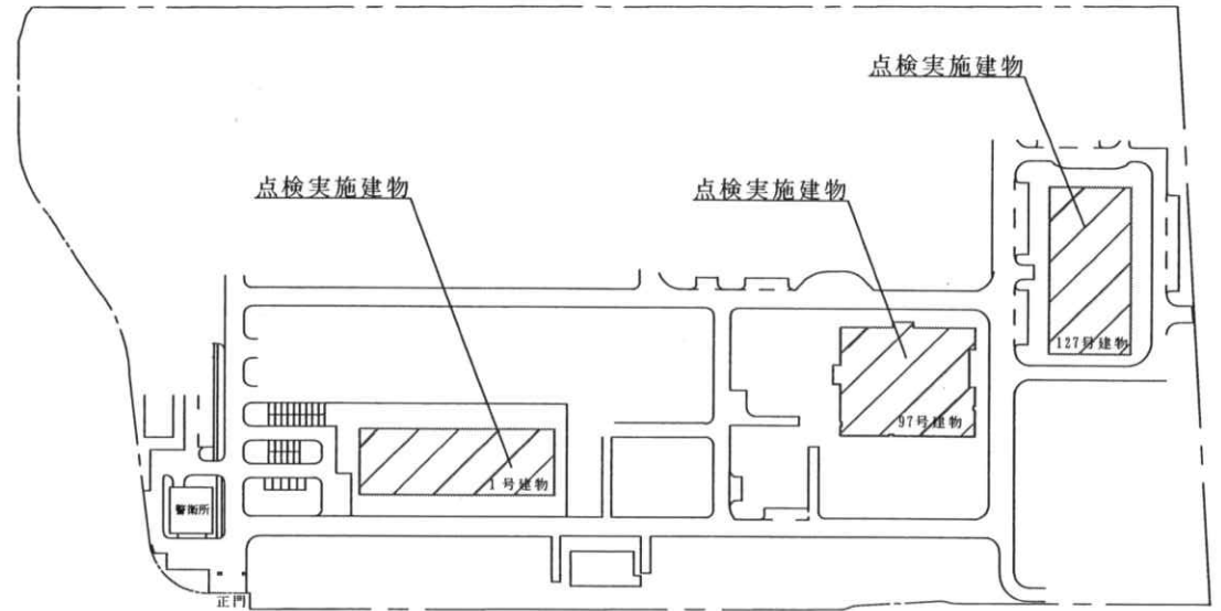
駐屯地配置図 S=1:2,000
