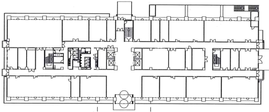
1号庁舎平面図 S = 1 : 1.5
