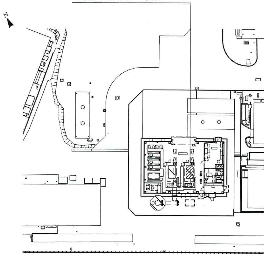
110号ボイラー室平面図 S=1/150
