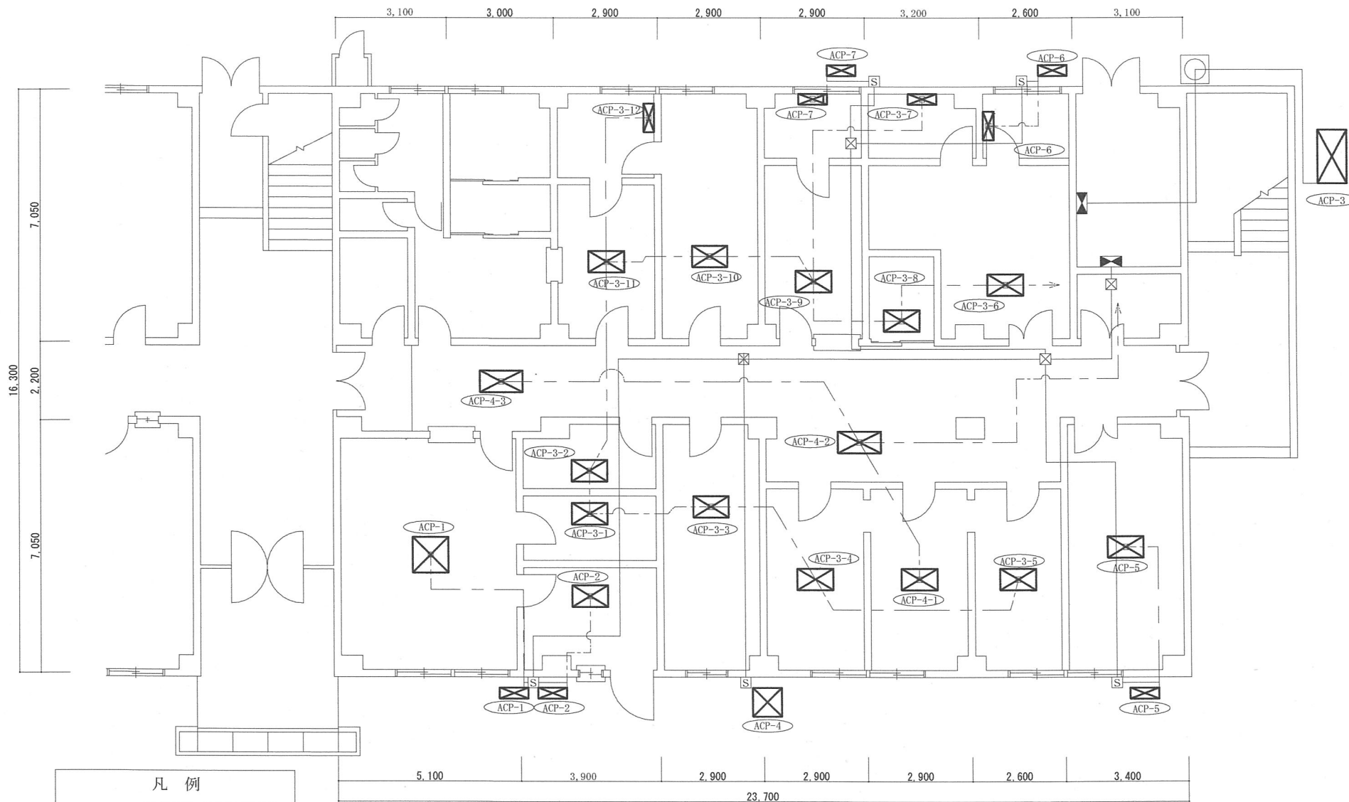
空調設備 (電源線) 詳細図 S=1/150
