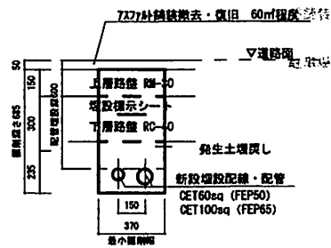
道路埋設断面図 (標準) S=1:20
