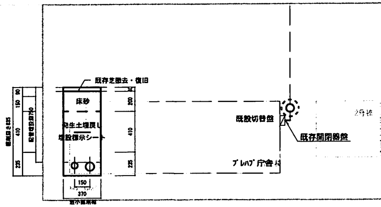
芝面埋設断面図 (標準) S=1:20
