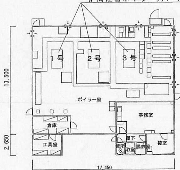
15号建物平面図 S=1/300
