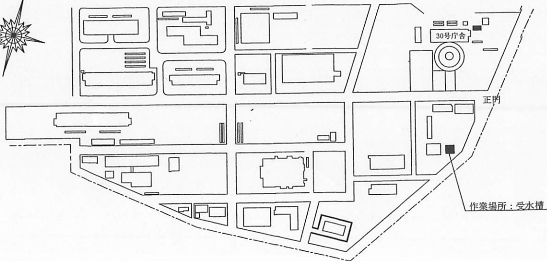
配置図 S=1/7000
