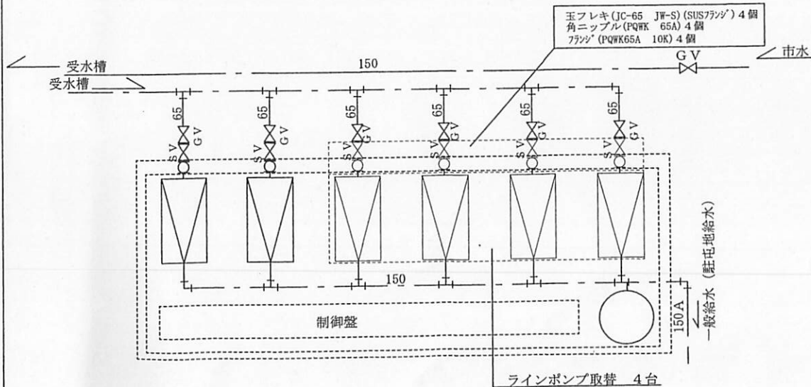
一般給水ユニット平面図
