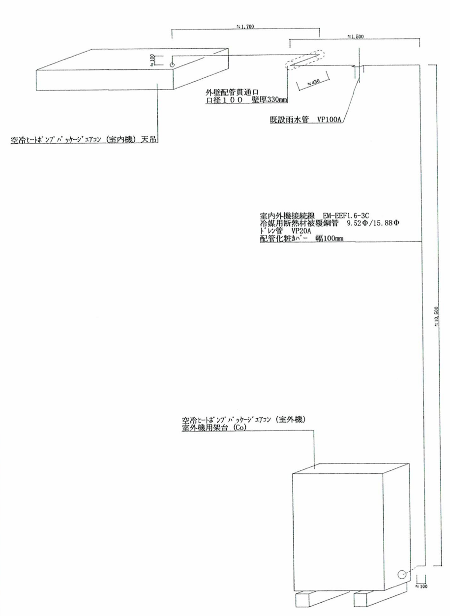
空調機設置標準立面図 (北面) S = 1 / X
