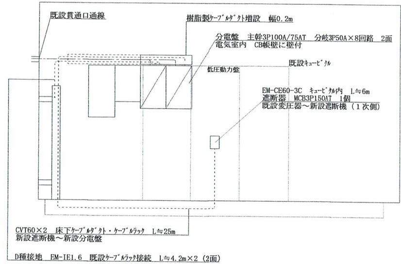
新設分電盤標準図 S=1/X
