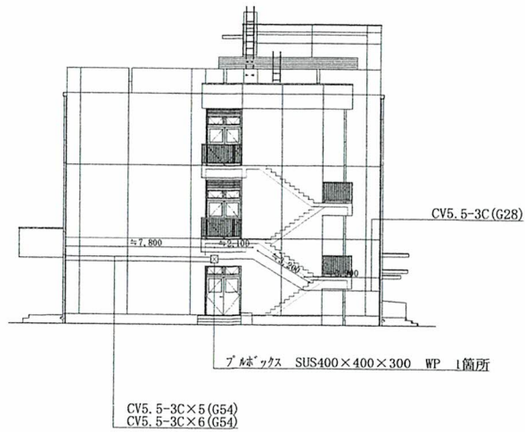
キュービクル改修図 S=1/X
