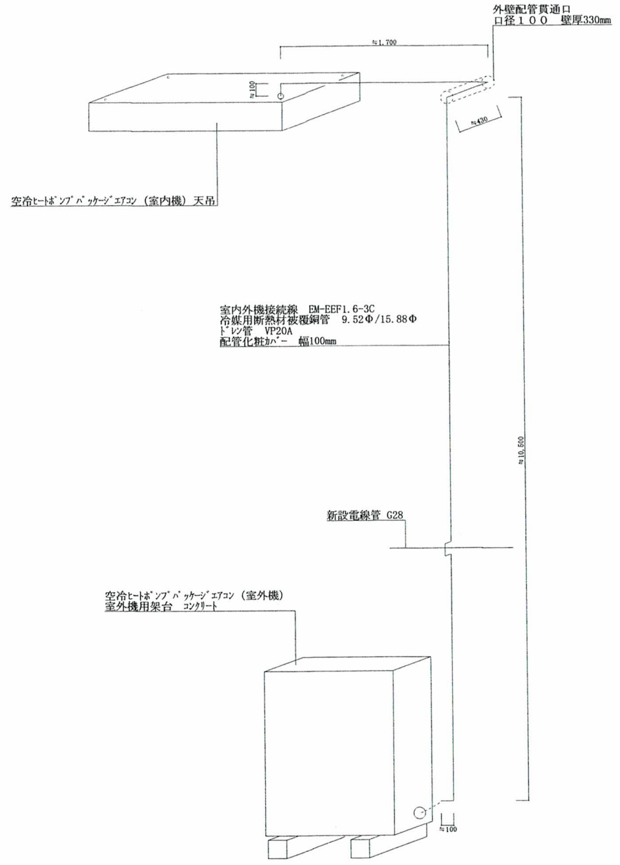
空調機設置標準立面図 (南面) S = 1 / X
