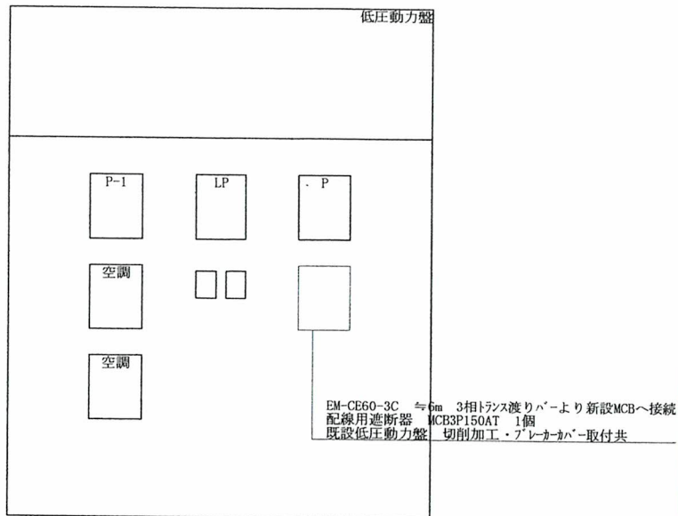
キュービクル改修図 S=1/X
