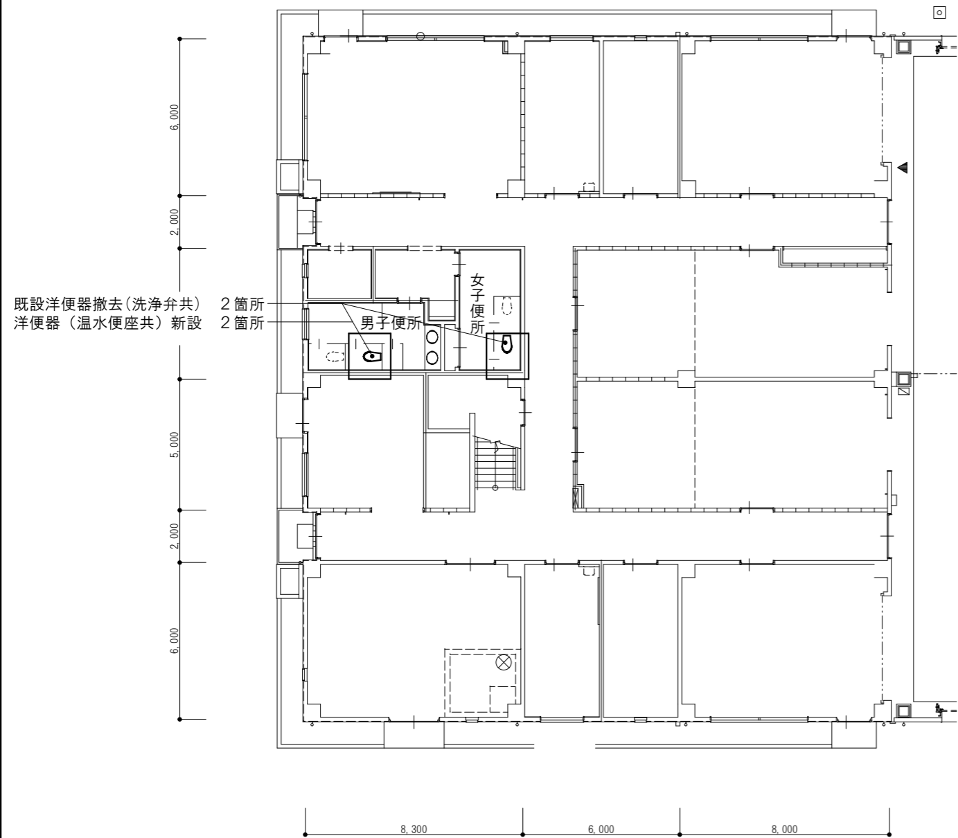
265号建物1階平面図
