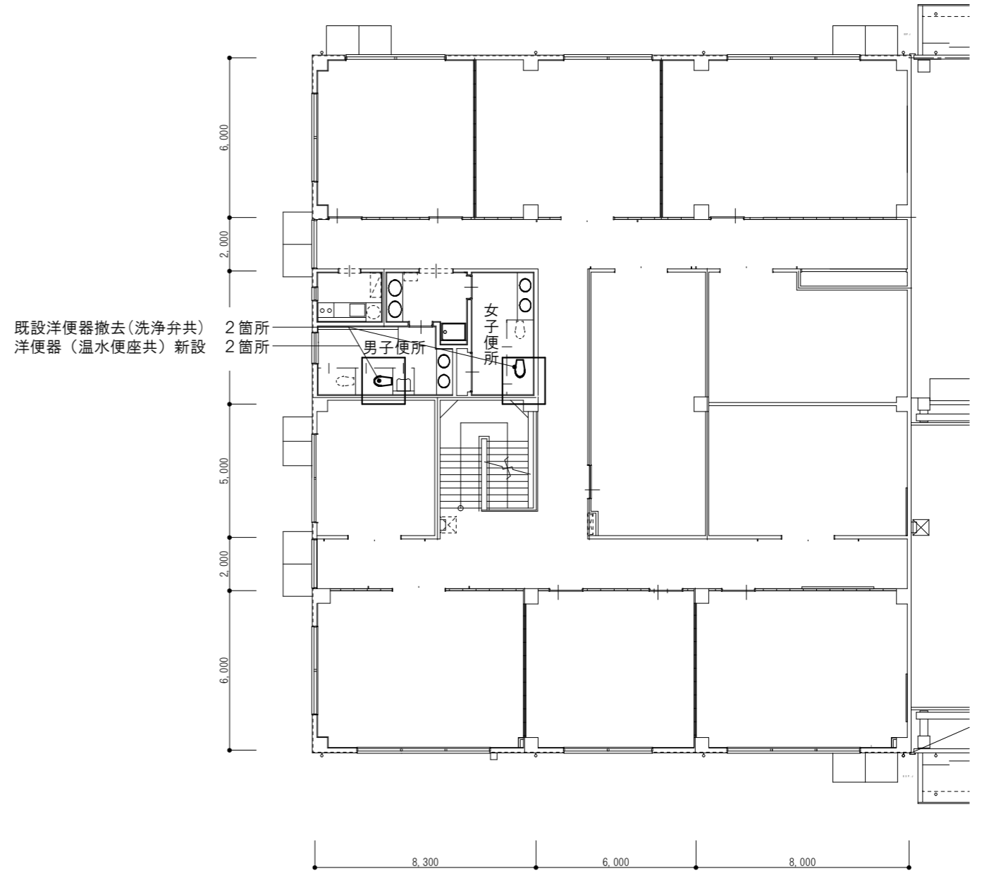
265号建物2階平面図
