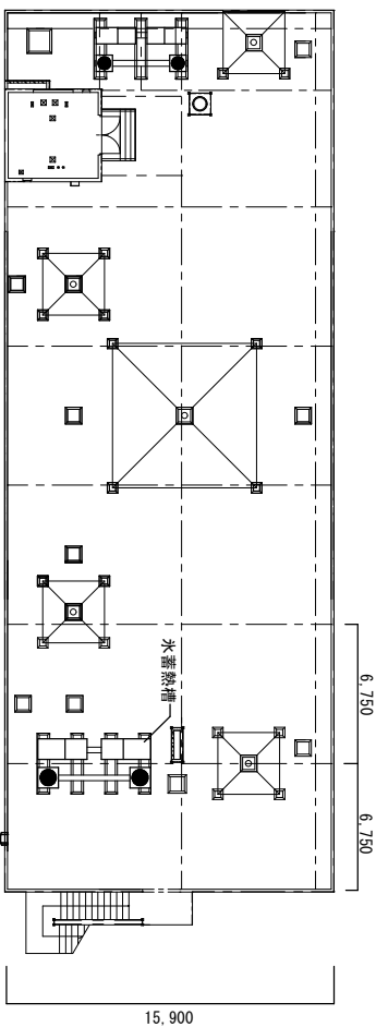
166号建物 RF 平面図 S=400
