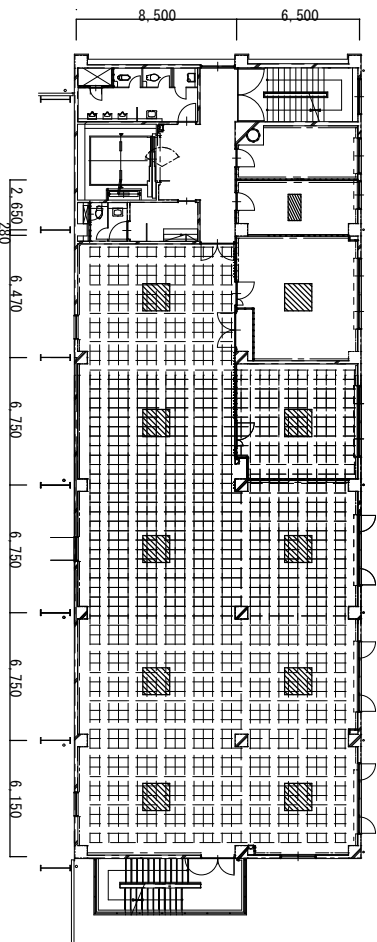
166号建物 3 F 平面図 S=400
