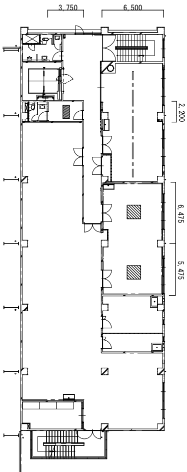
166号建物 2 F 平面図 S=400
