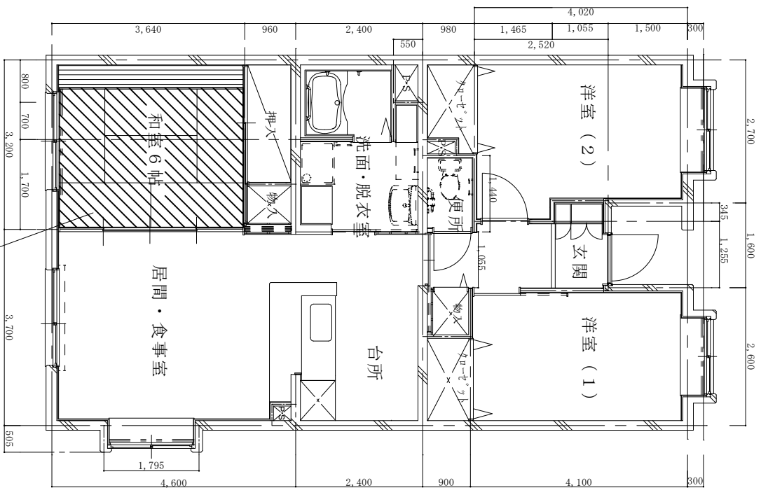
B棟201号室 平面図
