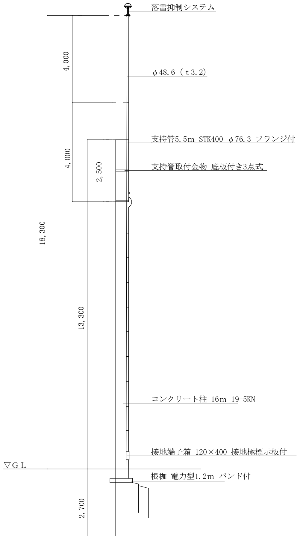
落雷抑制システム標準図 S=1/75
