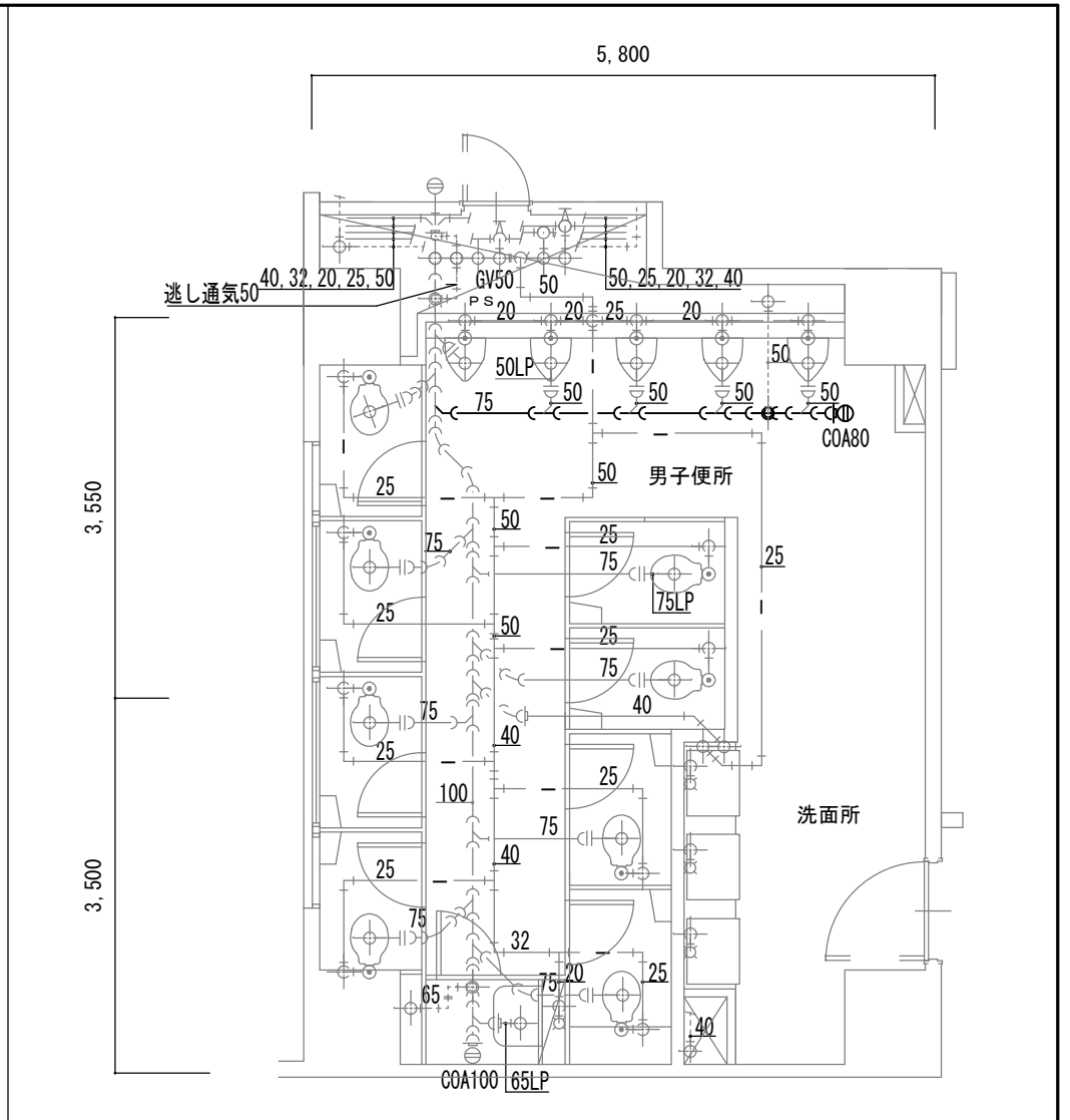
4～8階男子便所・洗面所詳細図 1/50
