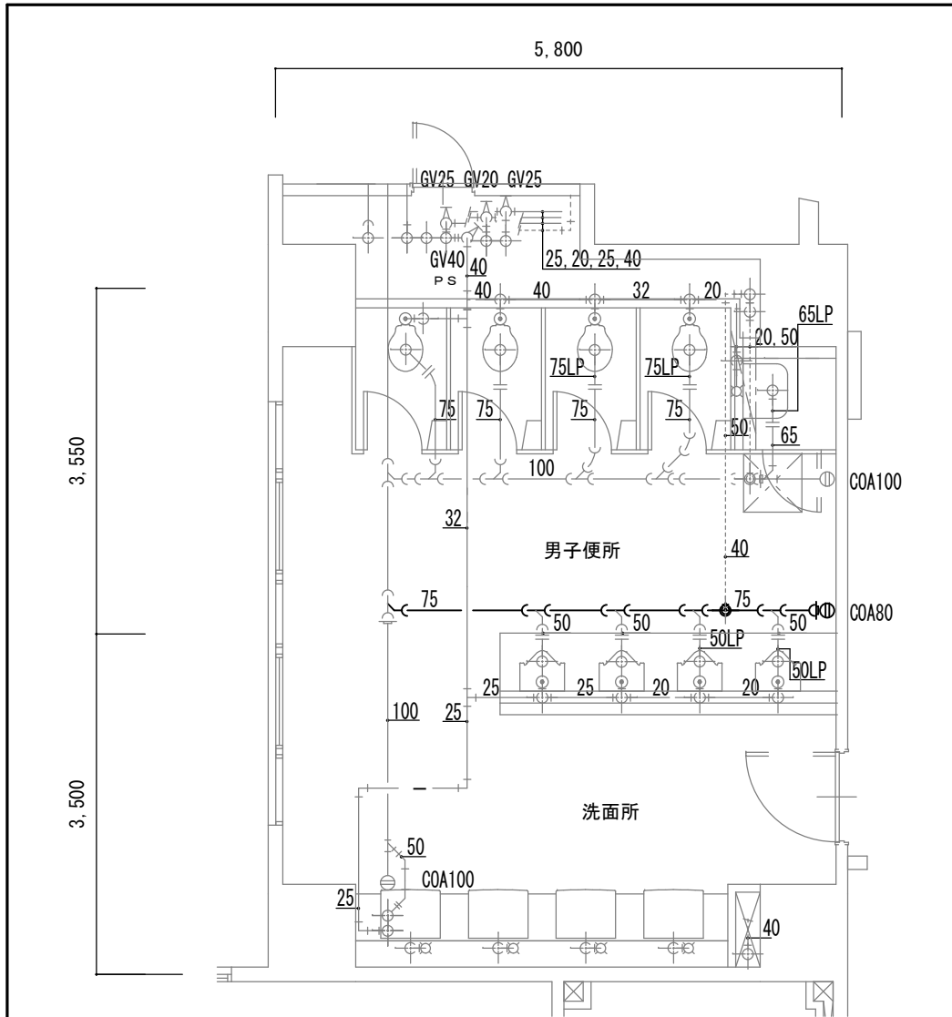
1～3階男子便所・洗面所詳細図 1/50
