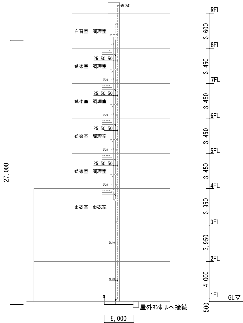
立配管図 1/X
