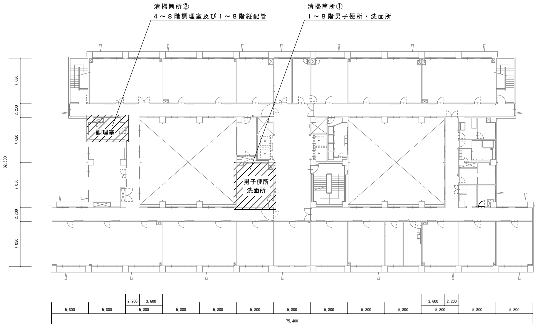
1号隊庁舎平面図 S=1/250
