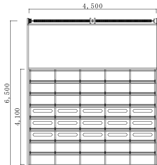
シャッター詳細図 1/75
