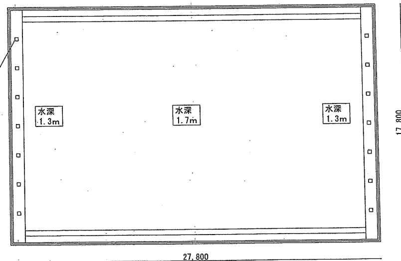
プール平面図 S=1/200
