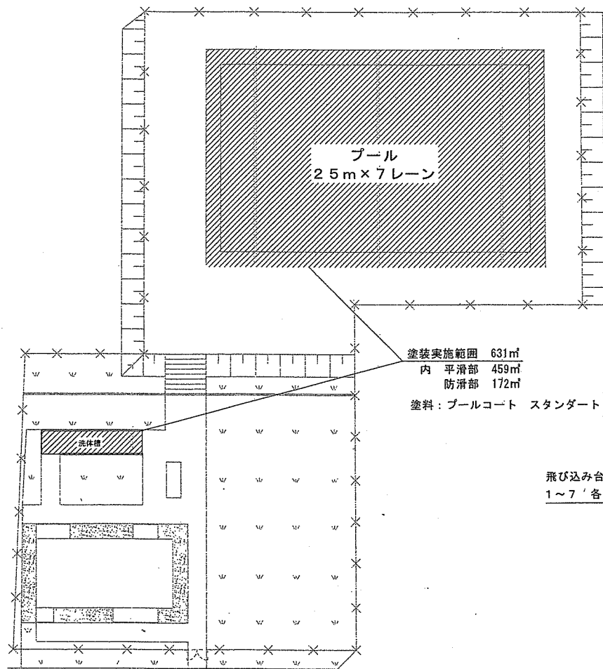
救命訓練場全体配置図 S=1/300
