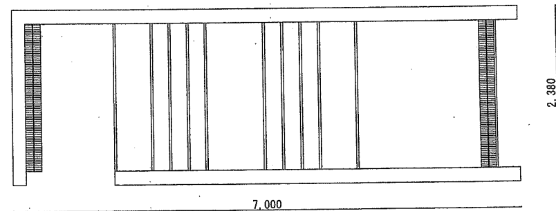
洗体槽平面図 S=1/50
