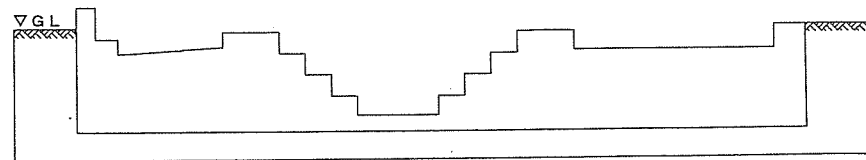
洗体槽断面図 S=1/50
