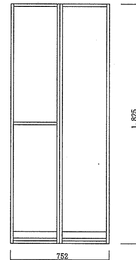
新設浴室折戸姿図 S=1/20
