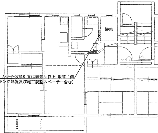
B棟505号室平面図 S=1/100
