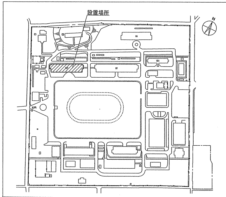
配置図 1:5,000
