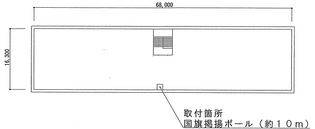
107号建物R階平面図 1:600
