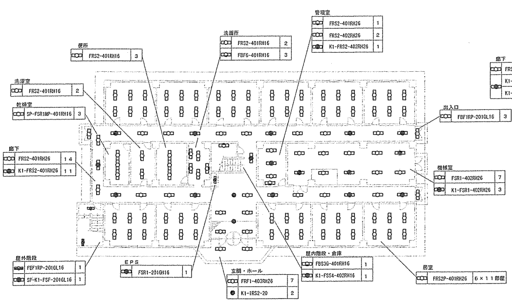
6号建物 1 F 電灯配置図 S=1/300
