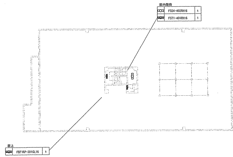
6号建物 R F 電灯配置図 S=1/300
