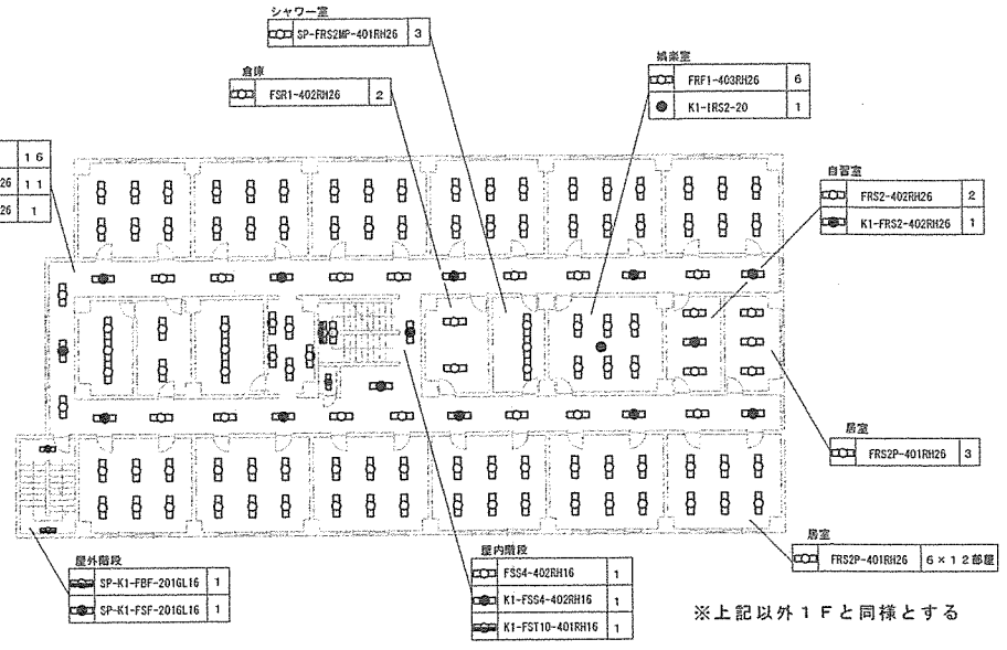
6号建物 4 F 電灯配置図 S=1/300
