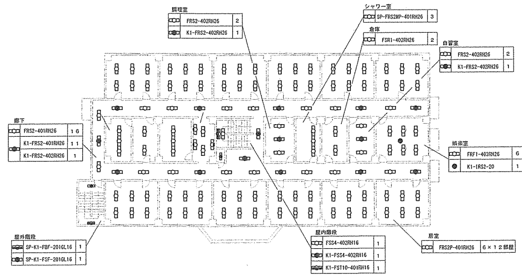
6号建物 2・3・5 F 電灯配置図 S=1/300
