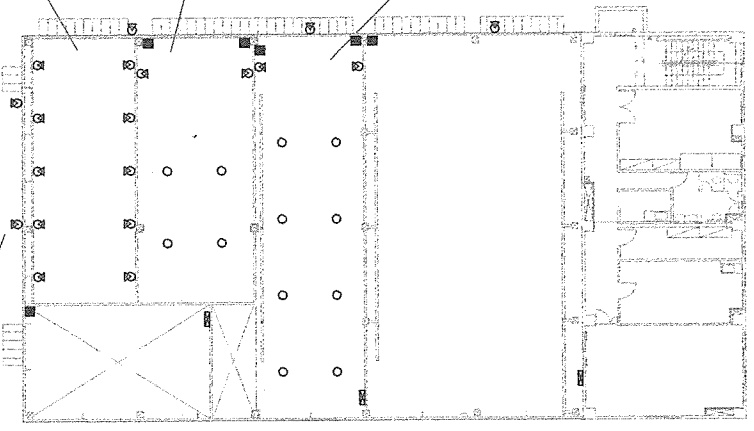
159号建物 2 F 電灯配置図 S=1/300
