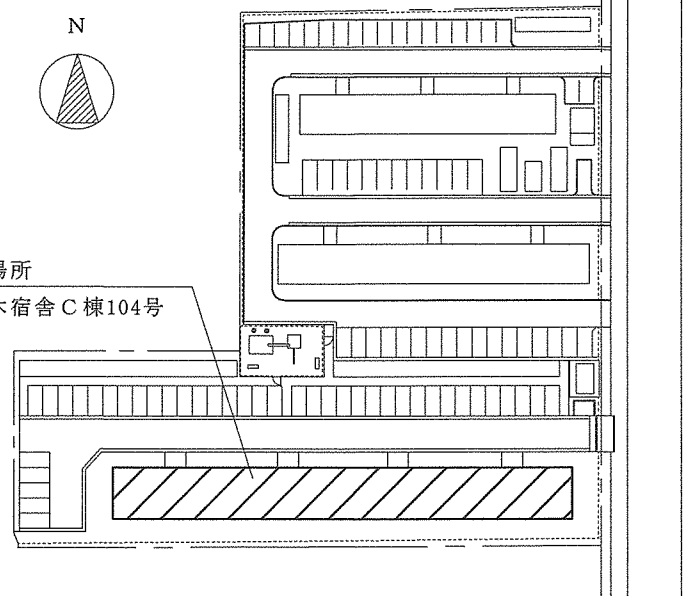
配置図 S=1:900
