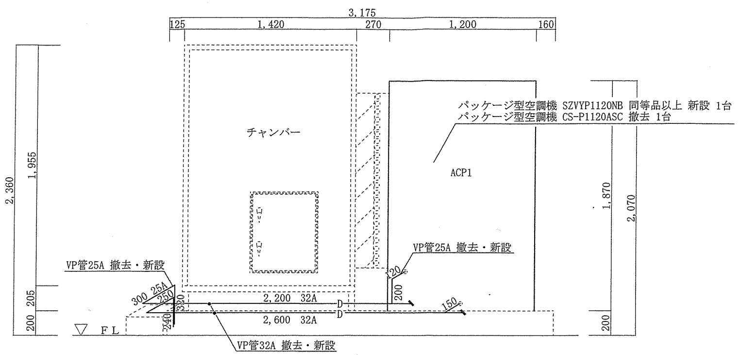
ACP1 D面立面図 S=1/30
