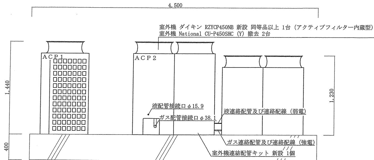
D面室外機立面図 S=1/20
