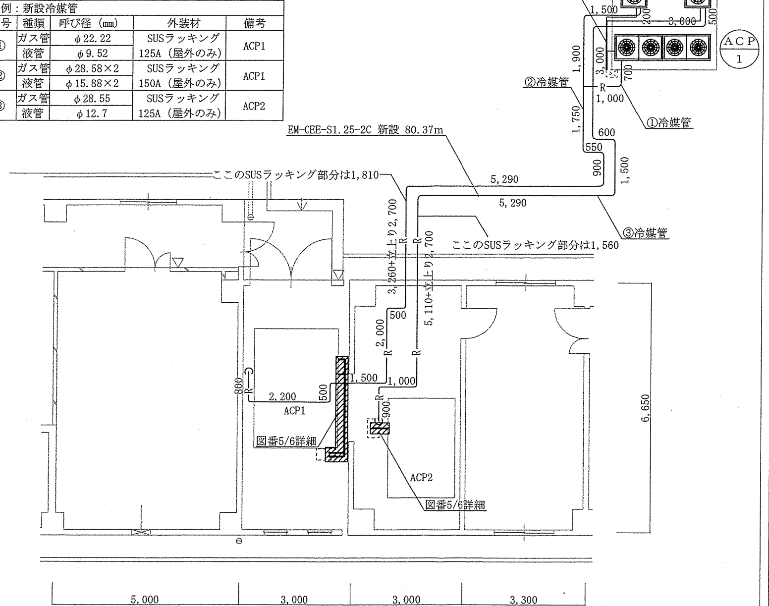
44号建物平面図 S=1/100
