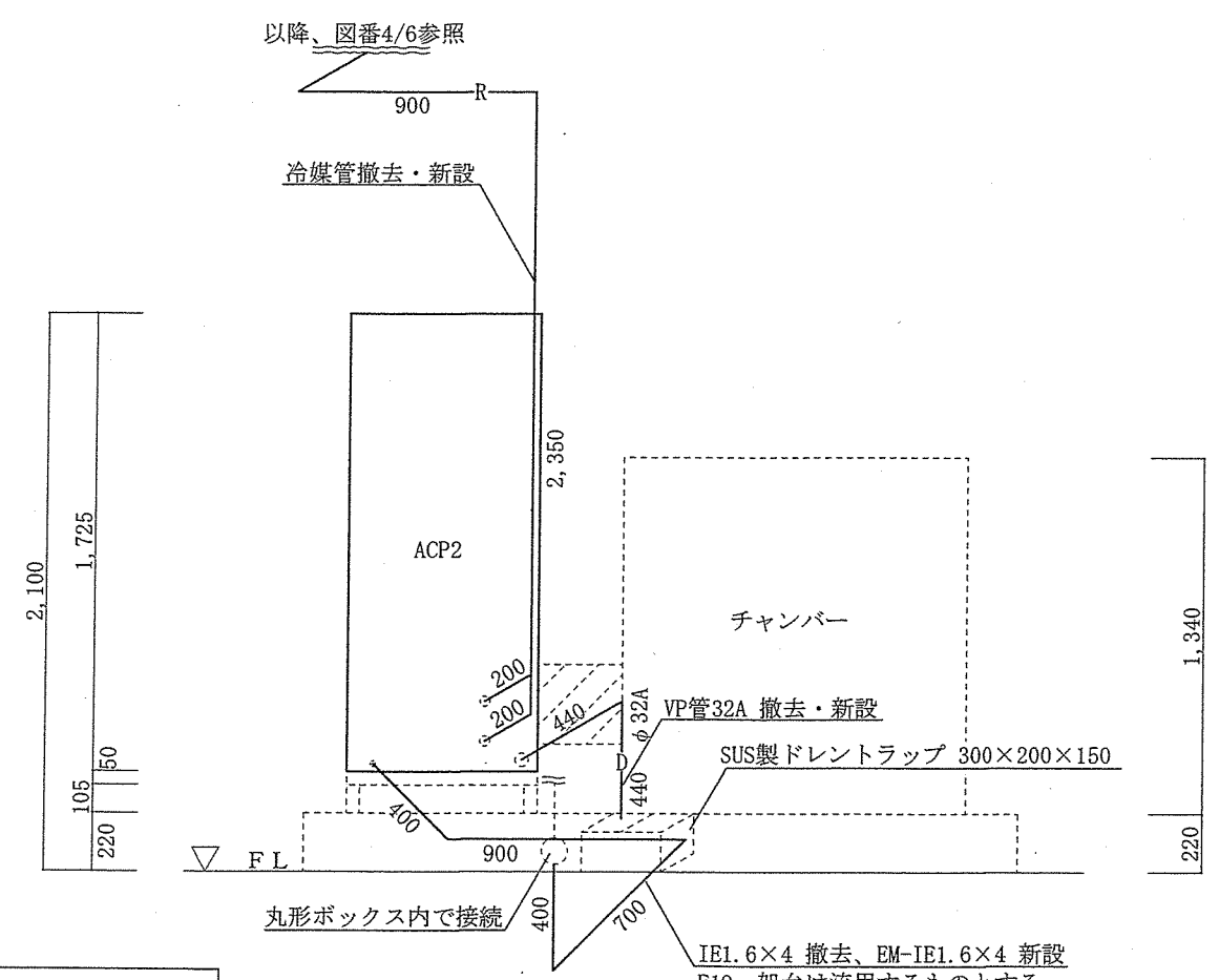
ACP2 B面立面図 S=1/30
