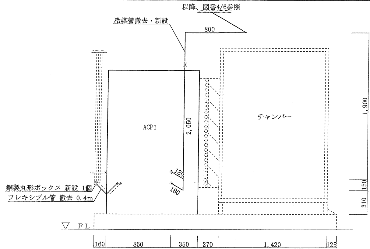
ACP1 B面立面図 S=1/30
