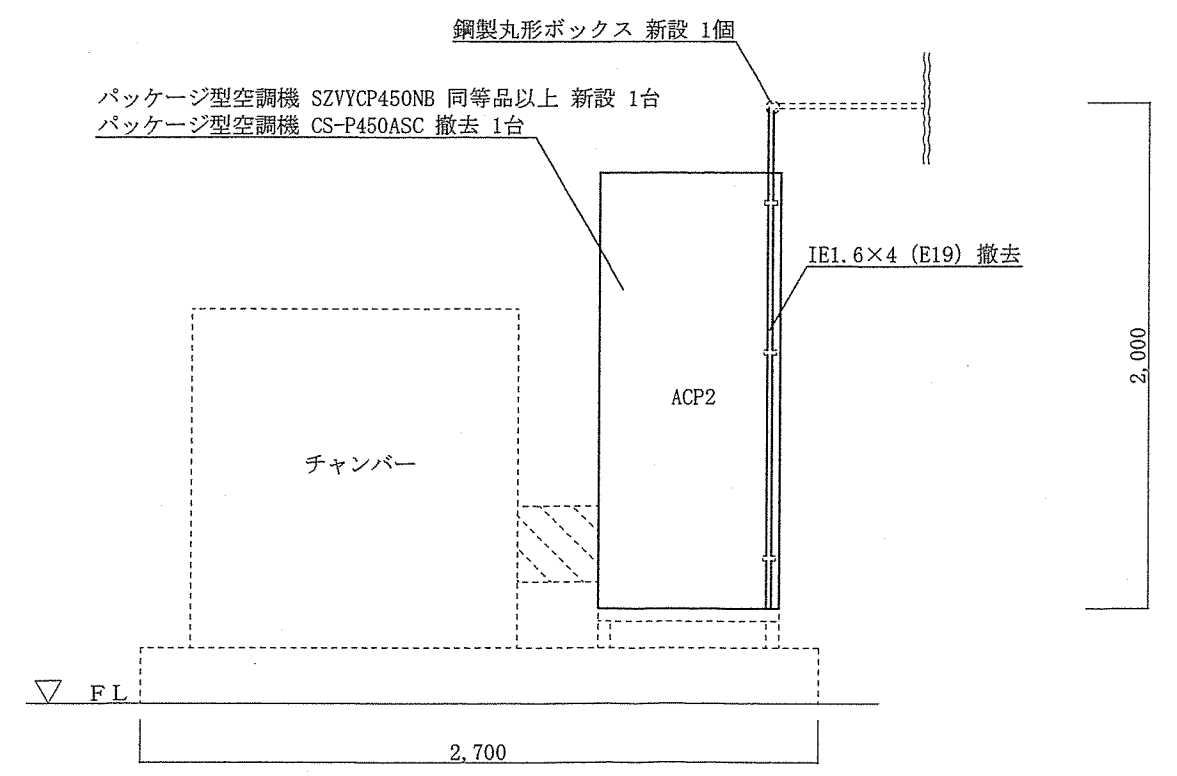
ACP2 D面立面図 S=1/30
