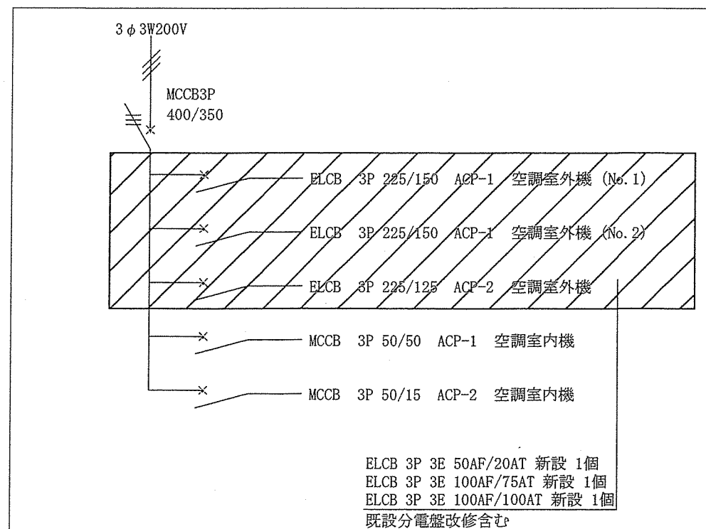
動力分電盤図 S=1/10
