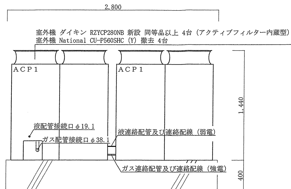
C面室外機立面図 S=1/20
