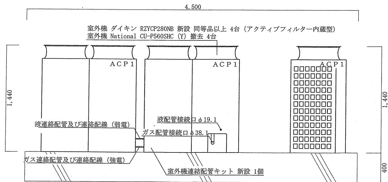
B面室外機立面図 S=1/20
