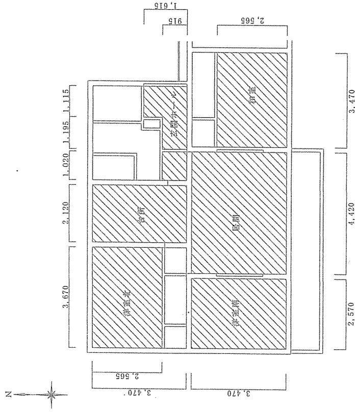
生野宿舍1棟d規格 天井伏せ図 S=1/100
