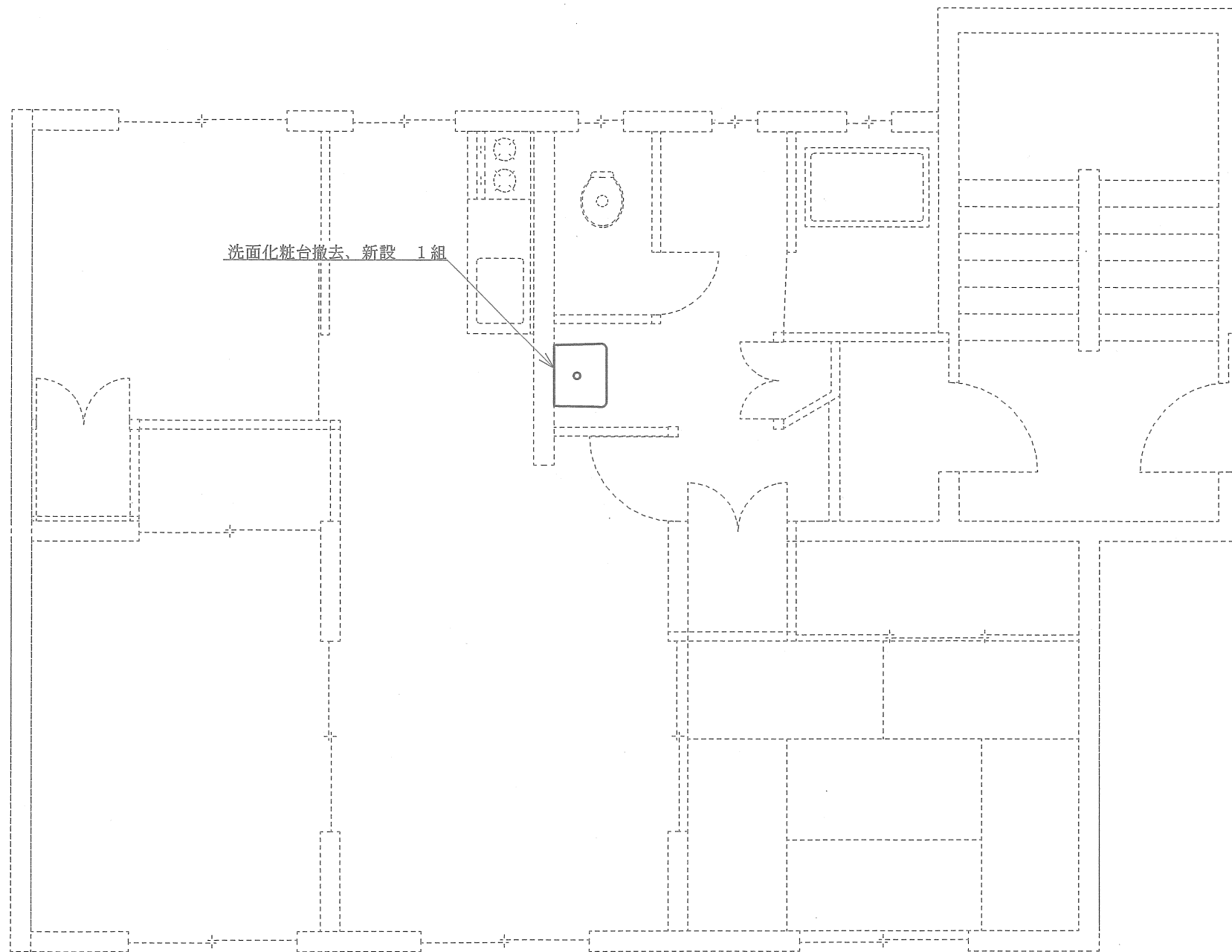
2・3号棟平面図 1/50
