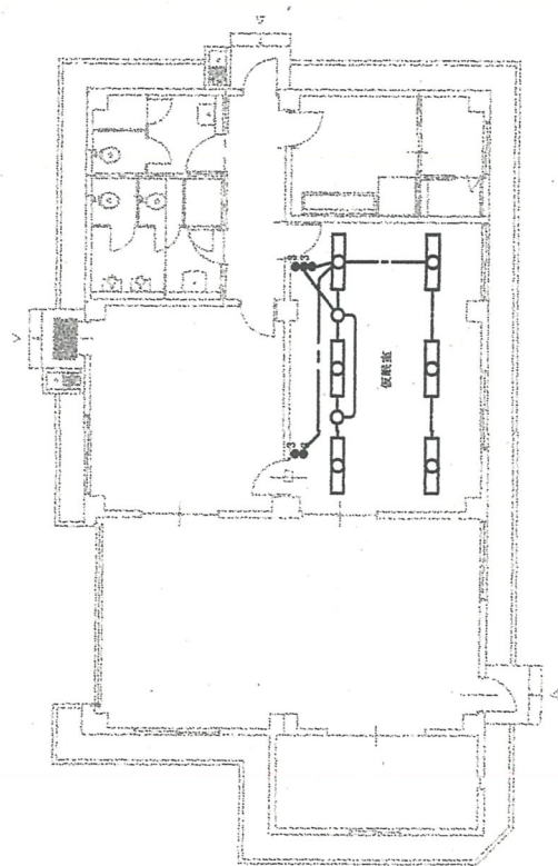
空調設備平面図 S=1/200
