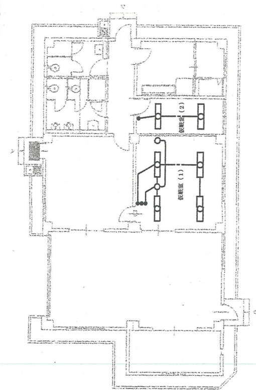
電源工事平面図 S=1/200
