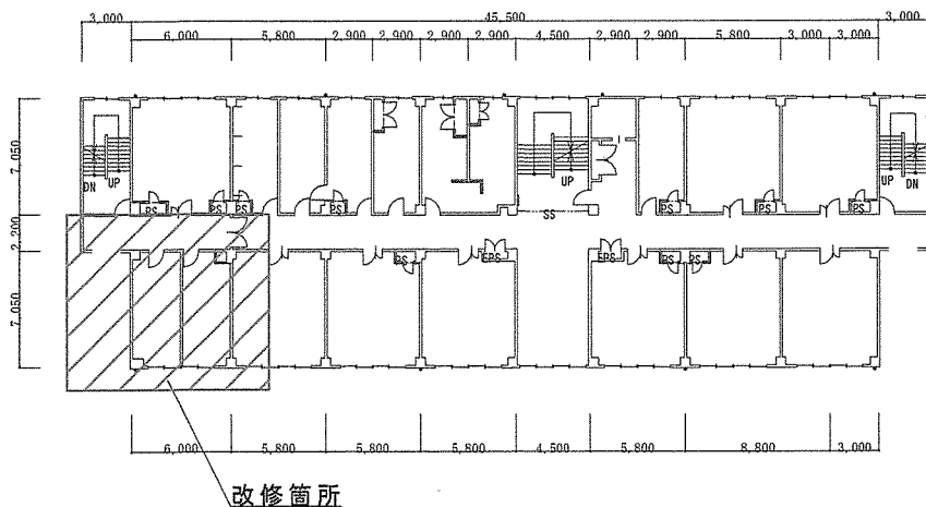
87号建物5階平面図 S=1:500
