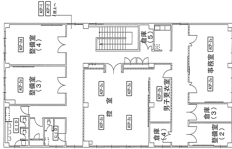
2階平面図
