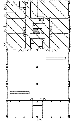
車両整備工場平面図
