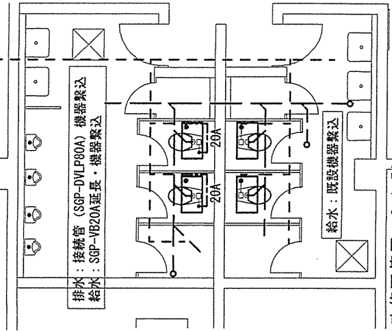
改修配管図 S=1:50
