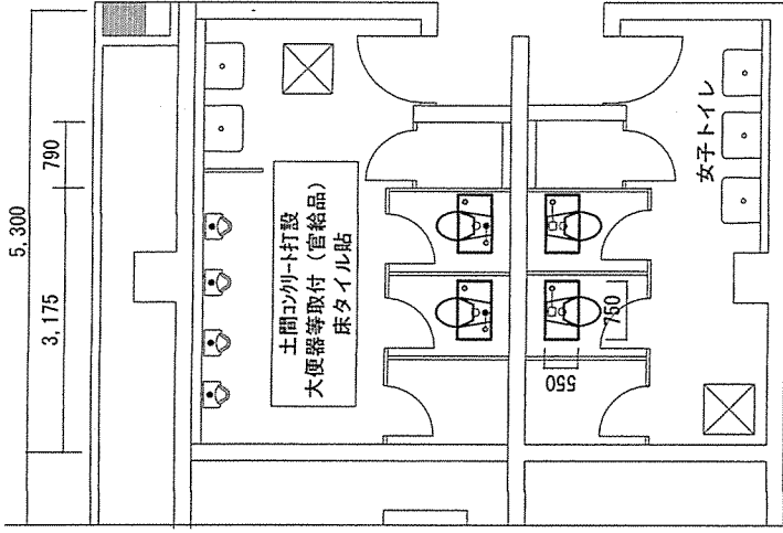
改修平面図 S=1:50
