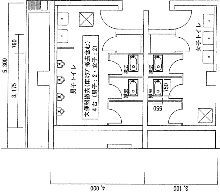
既設平面図 S=1:50
