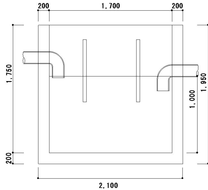
断面図
