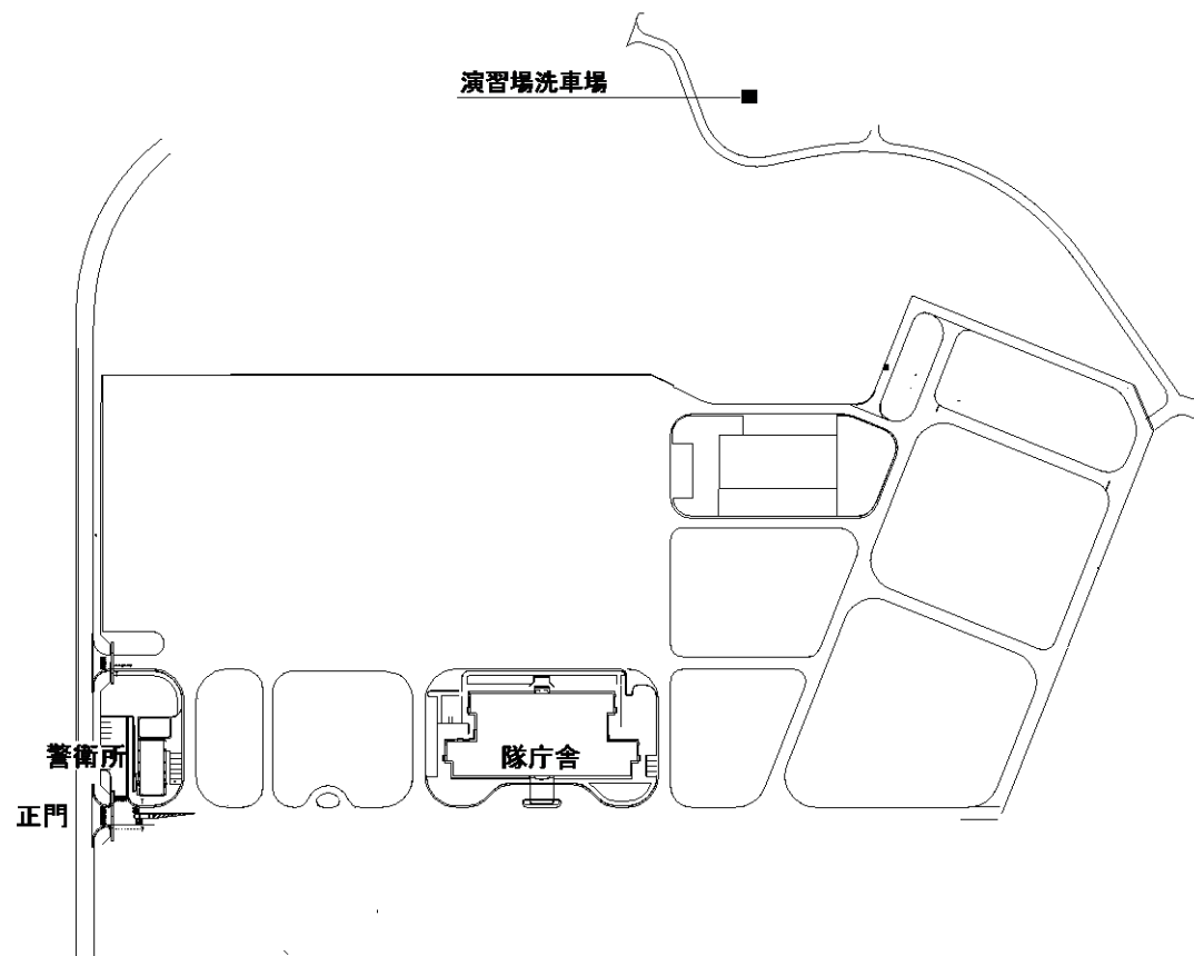
油分離槽配置図 S:1/4,000
