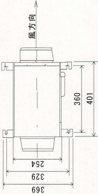
■外形図
