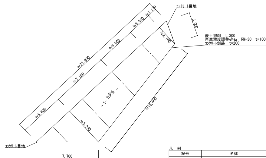
施工場所⑨改修平面図 S=1/200
