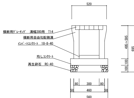
自由勾配側溝（横断面）断面図 S=1/20
