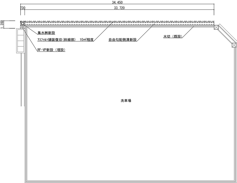
施工場所③洗車場平面図（改修後） S=1／250
