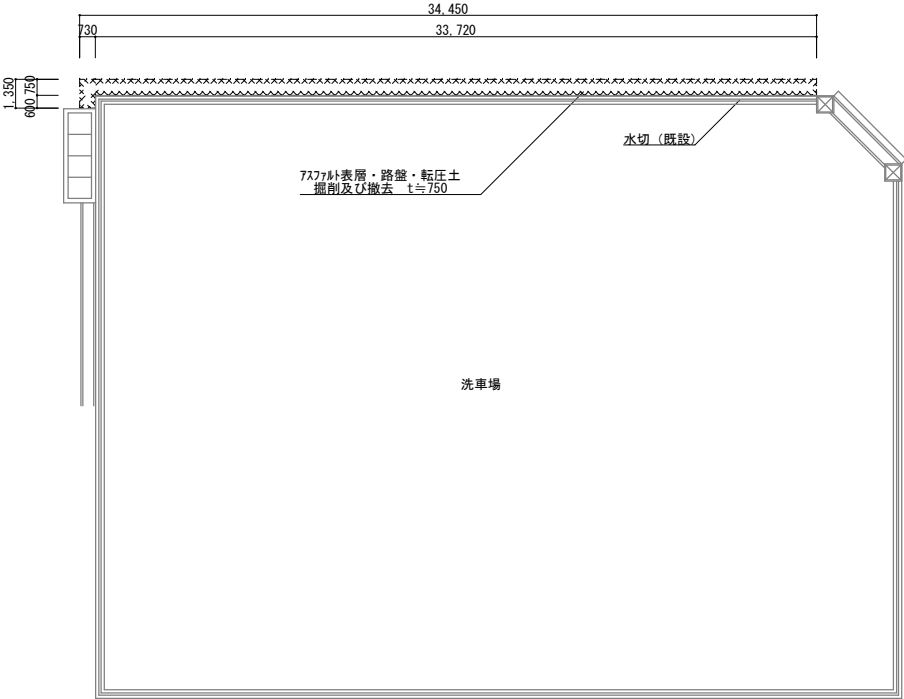
施工場所③洗車場平面図（改修前） S=1／250
