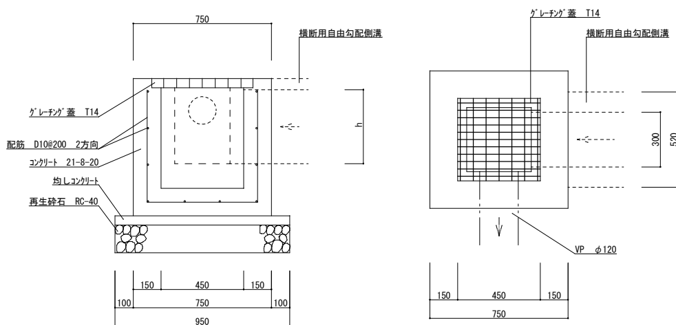
雨水枡断面図 S=1/20
