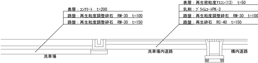
施工場所③洗車場周辺断面図（改修前） S=1／50
