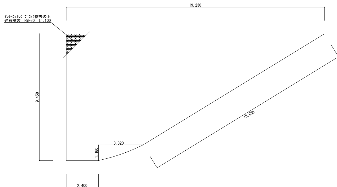
施工場所⑨改修平面図 S=1/200
