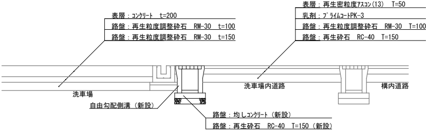
施工場所③洗車場周辺断面図（改修後） S=1／50
