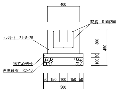
既設水切断面図 S=1/20
