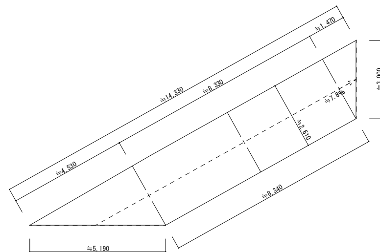
施工場所⑪改修平面図 S=1/100
