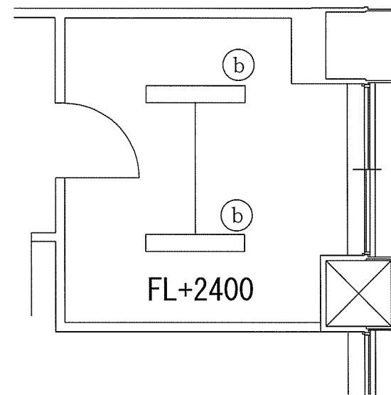
5 F 倉庫平面図
