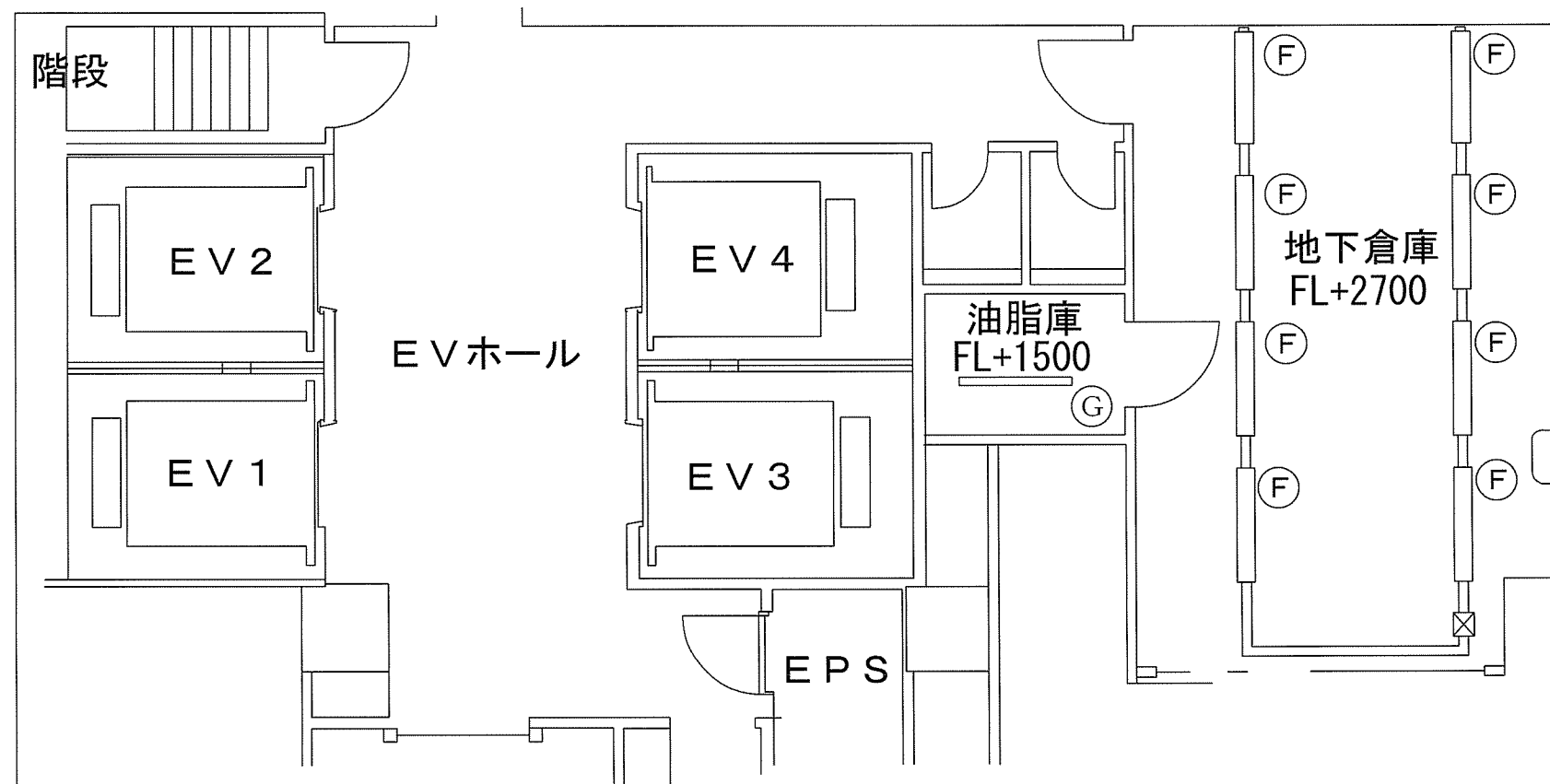
地下平面図
