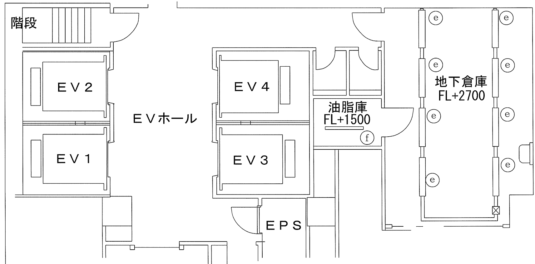
地下平面図
