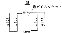
B部詳細図(埋込み部)
