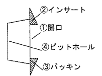
ピットホール取付詳細図
