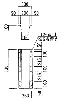
ピットホール SUS t=0.8
