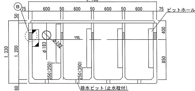
正面断面図
