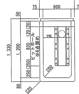
槽内断面図
