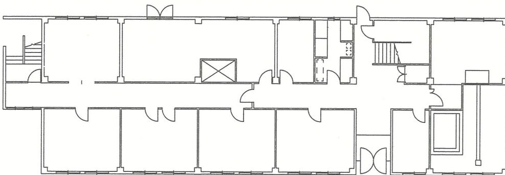
23号生活隊舎1階平面図
