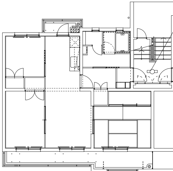
安芸宿舎標準平面図
