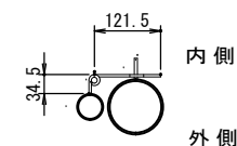
蝶番施錠詳細図
