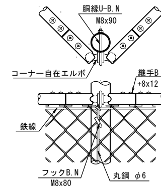
端柱取付詳細 (コーナー自在エルボ)
