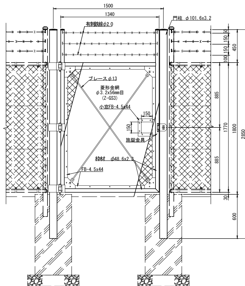
片開き門扉詳細図 S : 1/20
