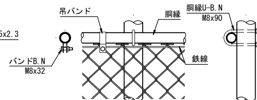
胴縁取付詳細
