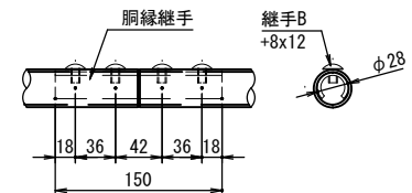
胴縁継手取付詳細
