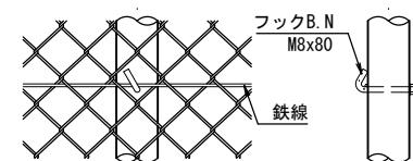
鉄線取付詳細
