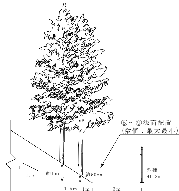
A-A' 法面樹木配置図
