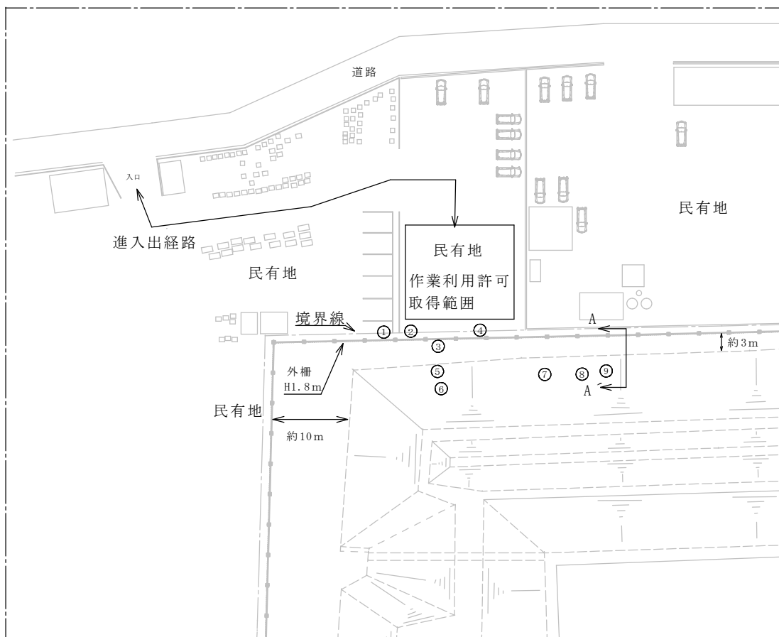
樹木周辺詳細図 S= 1 / X
