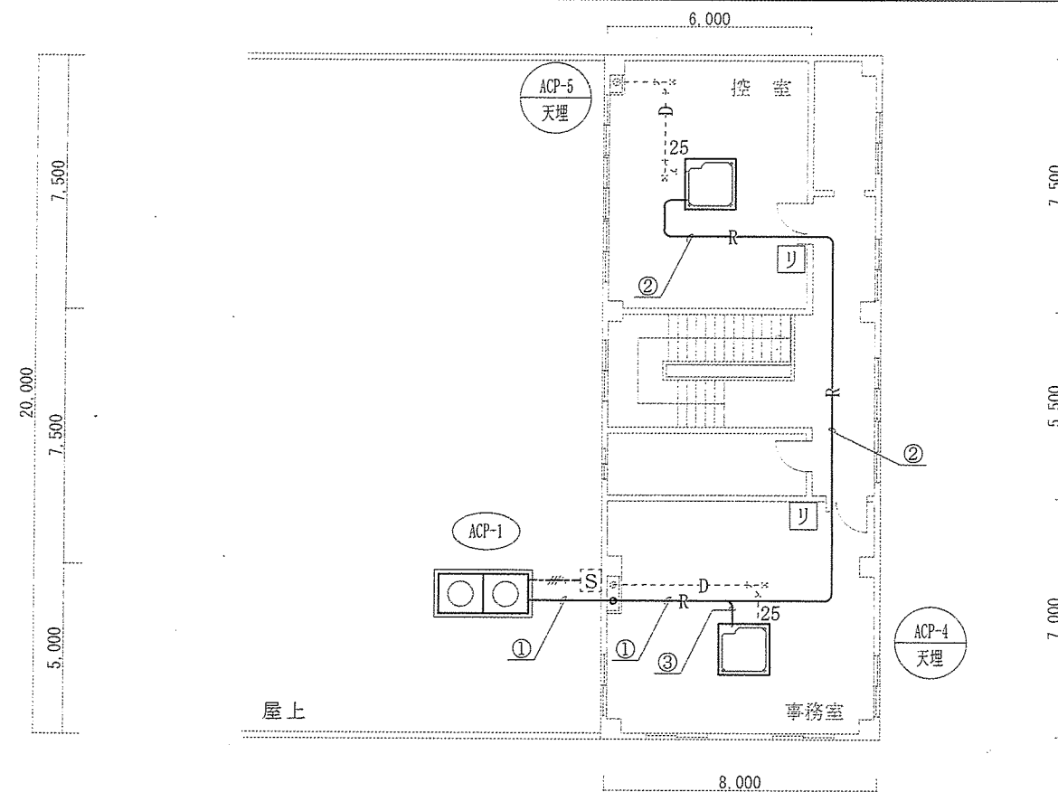
132号車両整備実習場 2階空調設備図 1:200
