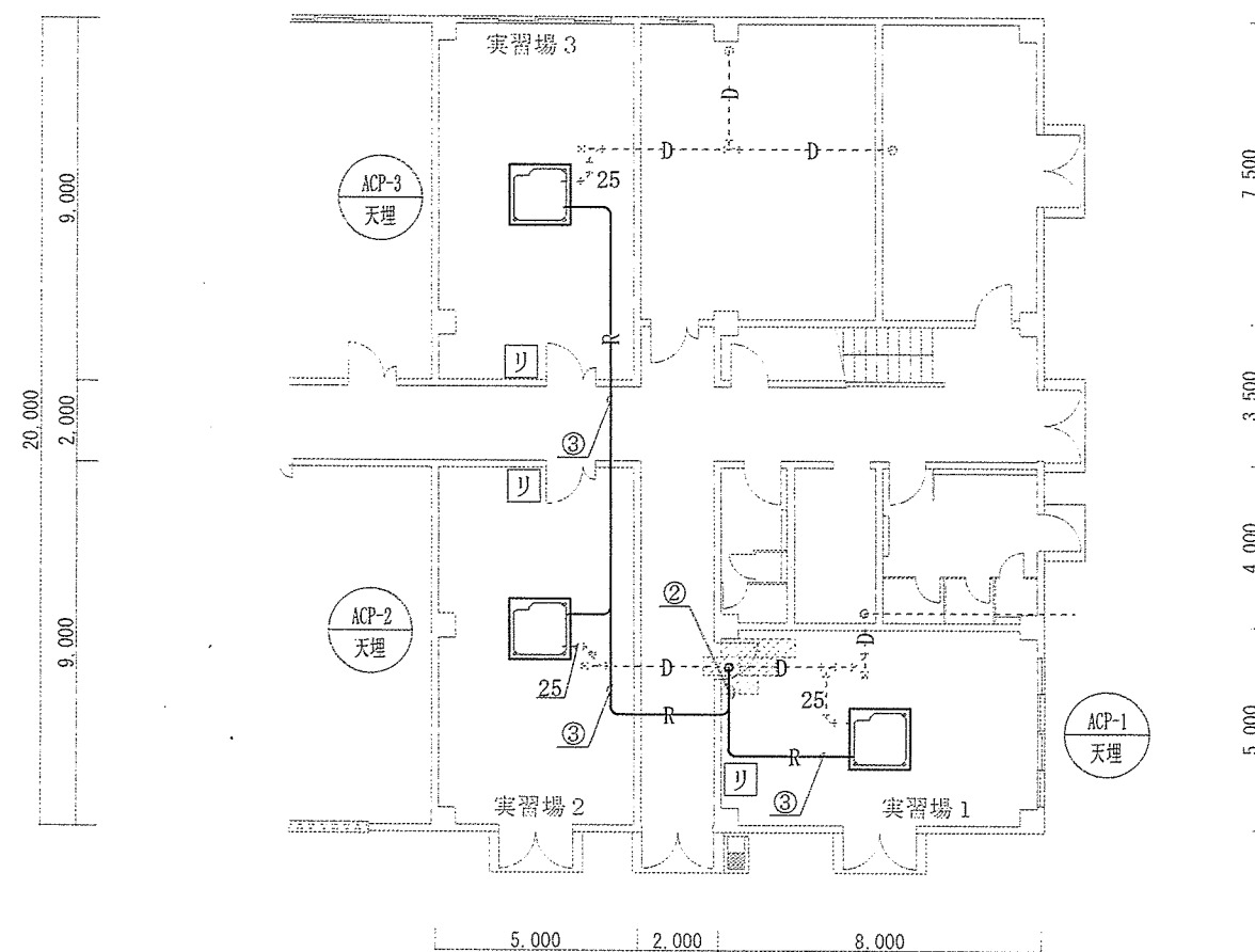
132号車両整備実習場 1階空調設備図 1:200
