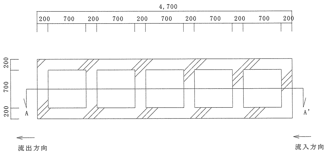
洗車場油分離槽平面図 S=1/40
