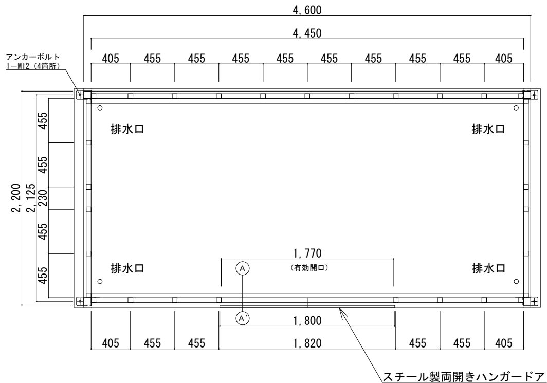
平面図 S=1/40
