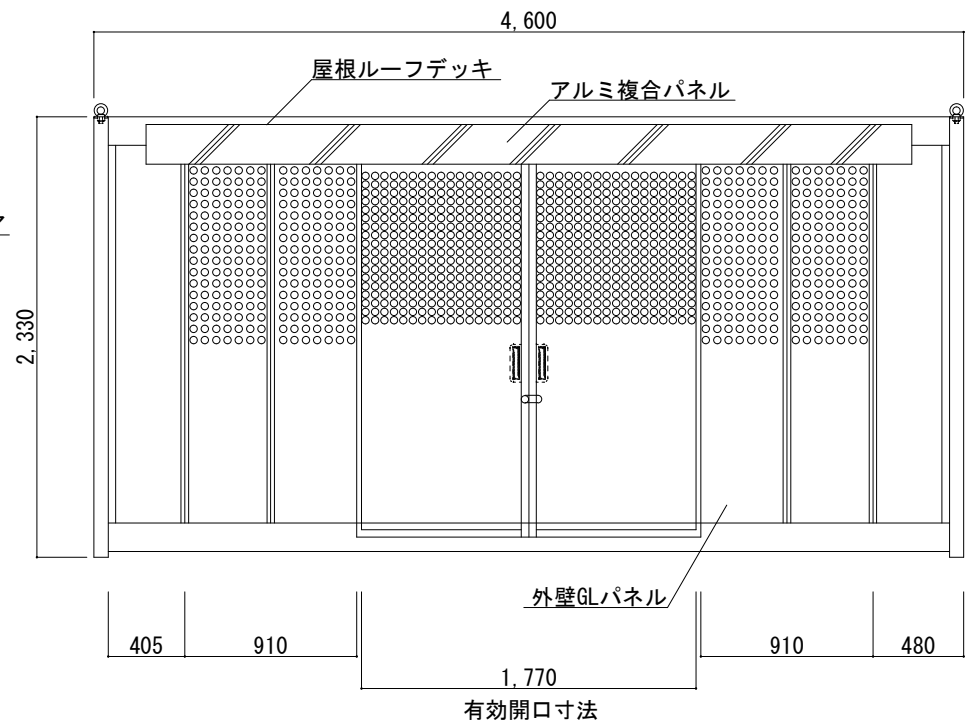
立面図 S=1/40
