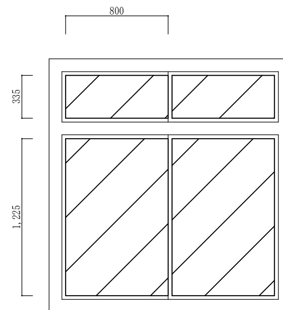
68号建物 10箇所 遮熱フィルム(3M NANO40S 同等品以上)貼付 鍛錬場
