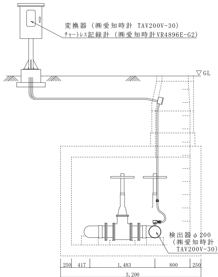
電磁流量計ピット断面図 S=1 : 30
