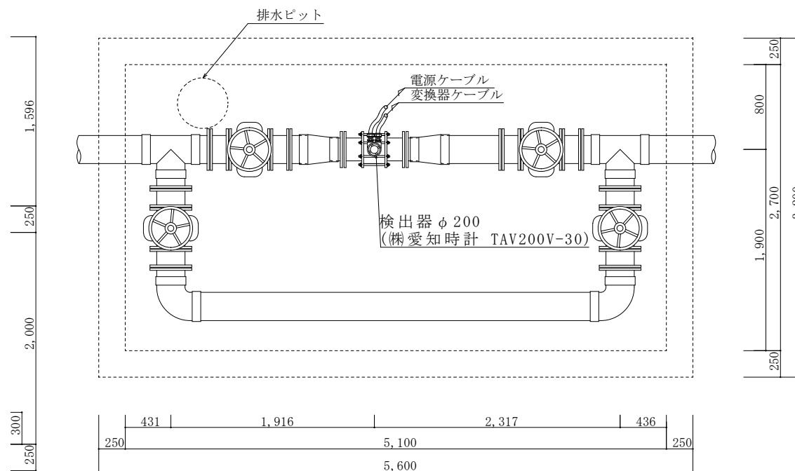
電磁流量計ピット内部平面図 S=1:30
