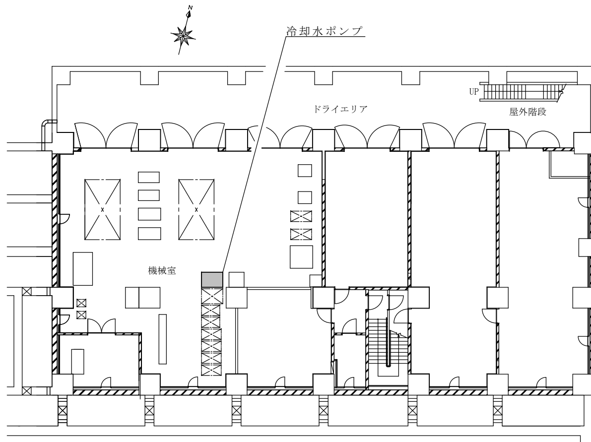
1号建物地階平面図 S = 1 / 2 5 0
