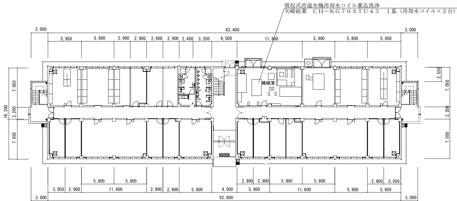
2号建物 1 階平面図 S=1:400
