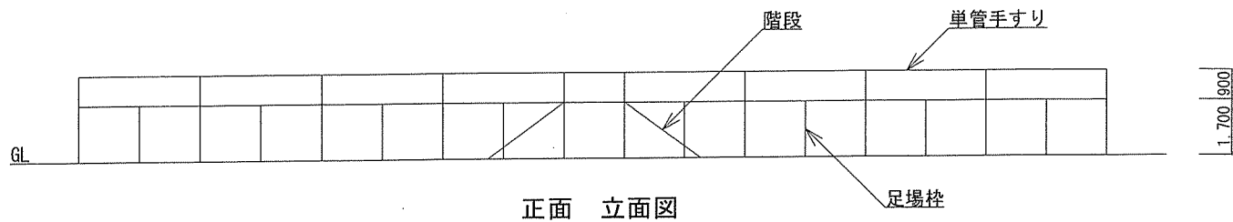
足場組立計画図（基準）
