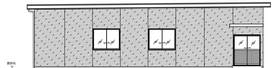
X0通り 立面図 S=1/100
