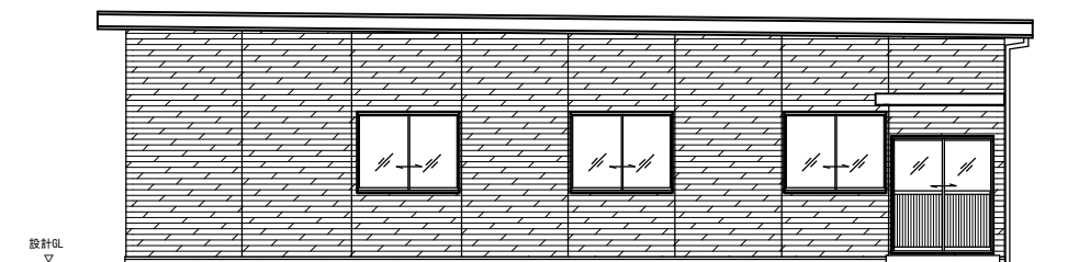
X14通り 立面図 S=1/100
