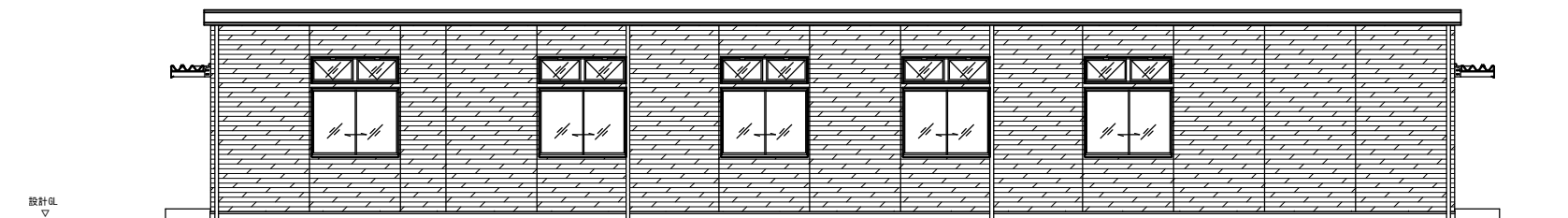
Y8通り 立面図 S=1/100
