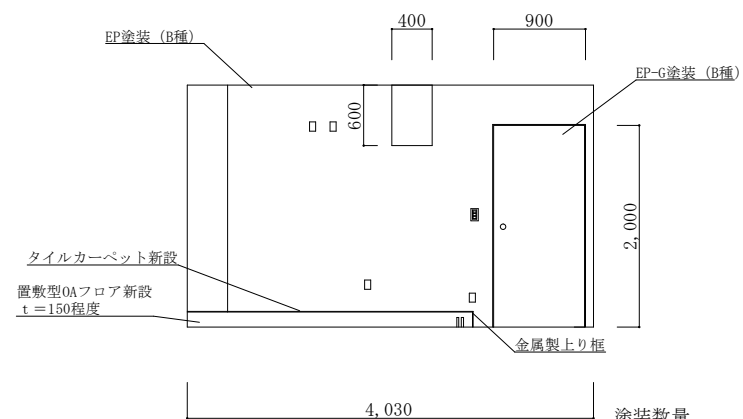
改修D面展開図
