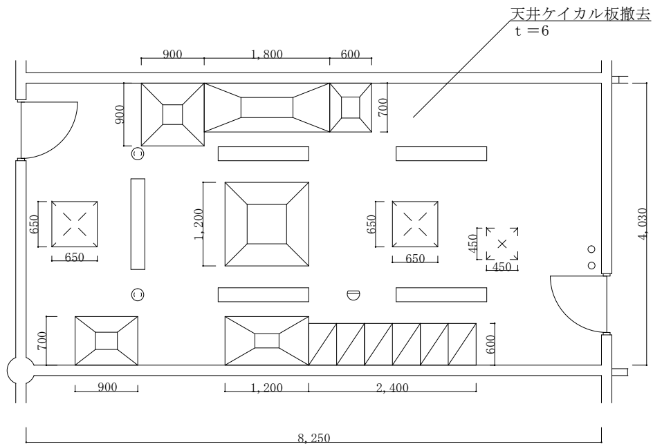
既設天井伏図
