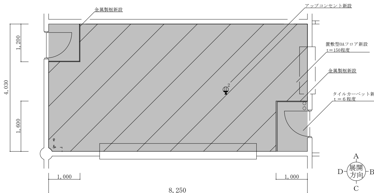
改修平面図
