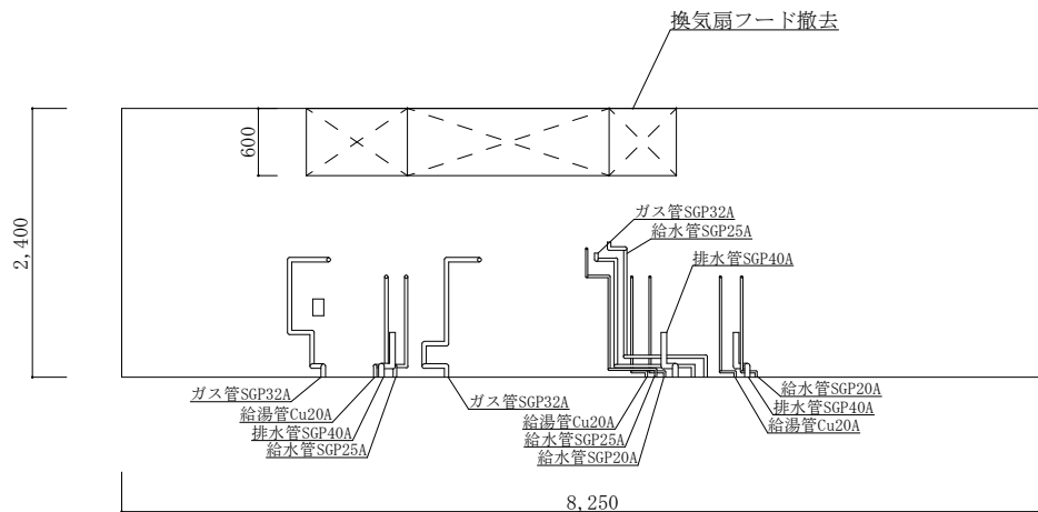
既設A面展開図
