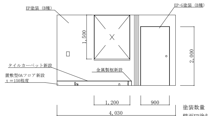
改修B面平面図
