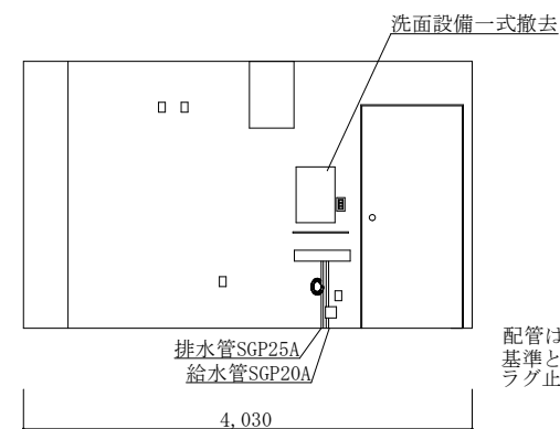
既設面D展開図
