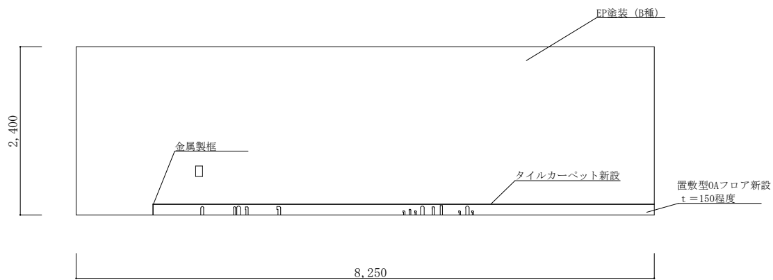
改修A面平面図
