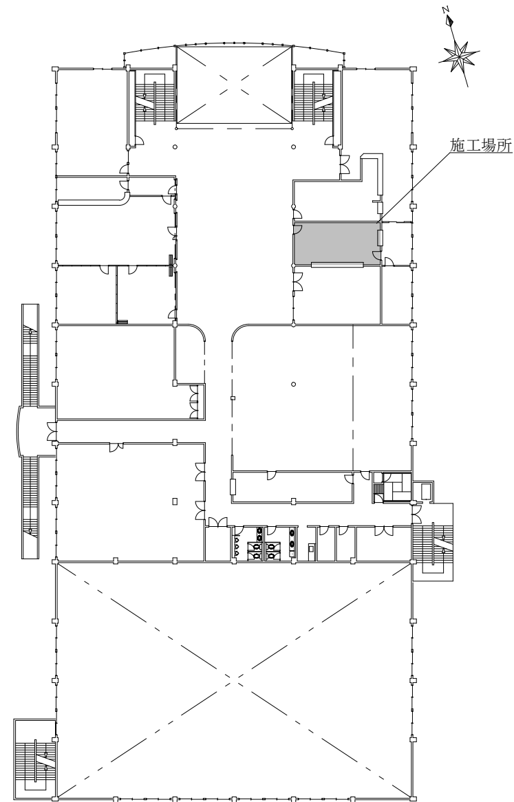
127号建物2F平面図 S=1:500
