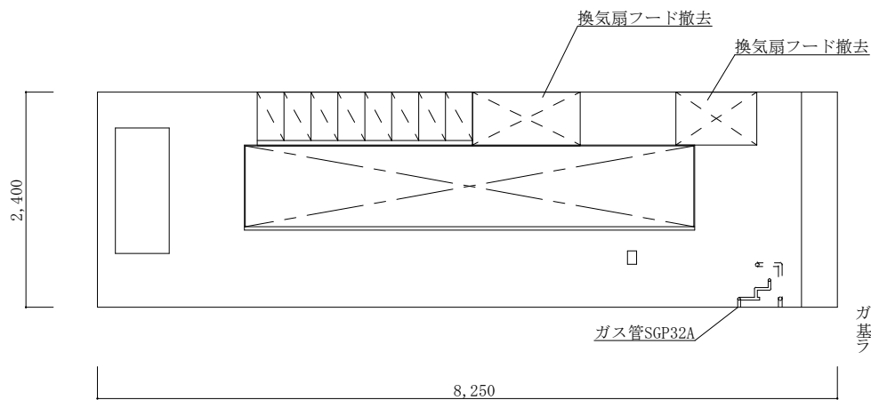
既設C面展開図
