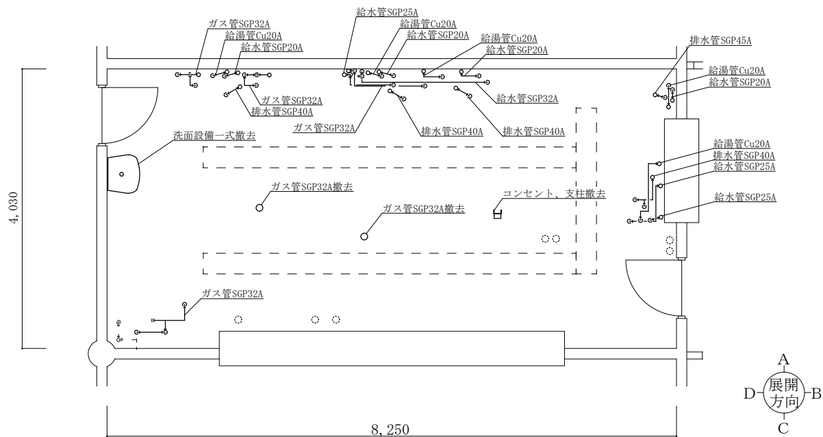
既設平面図
