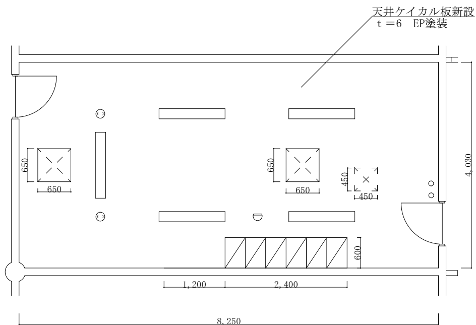
改修天井伏図
