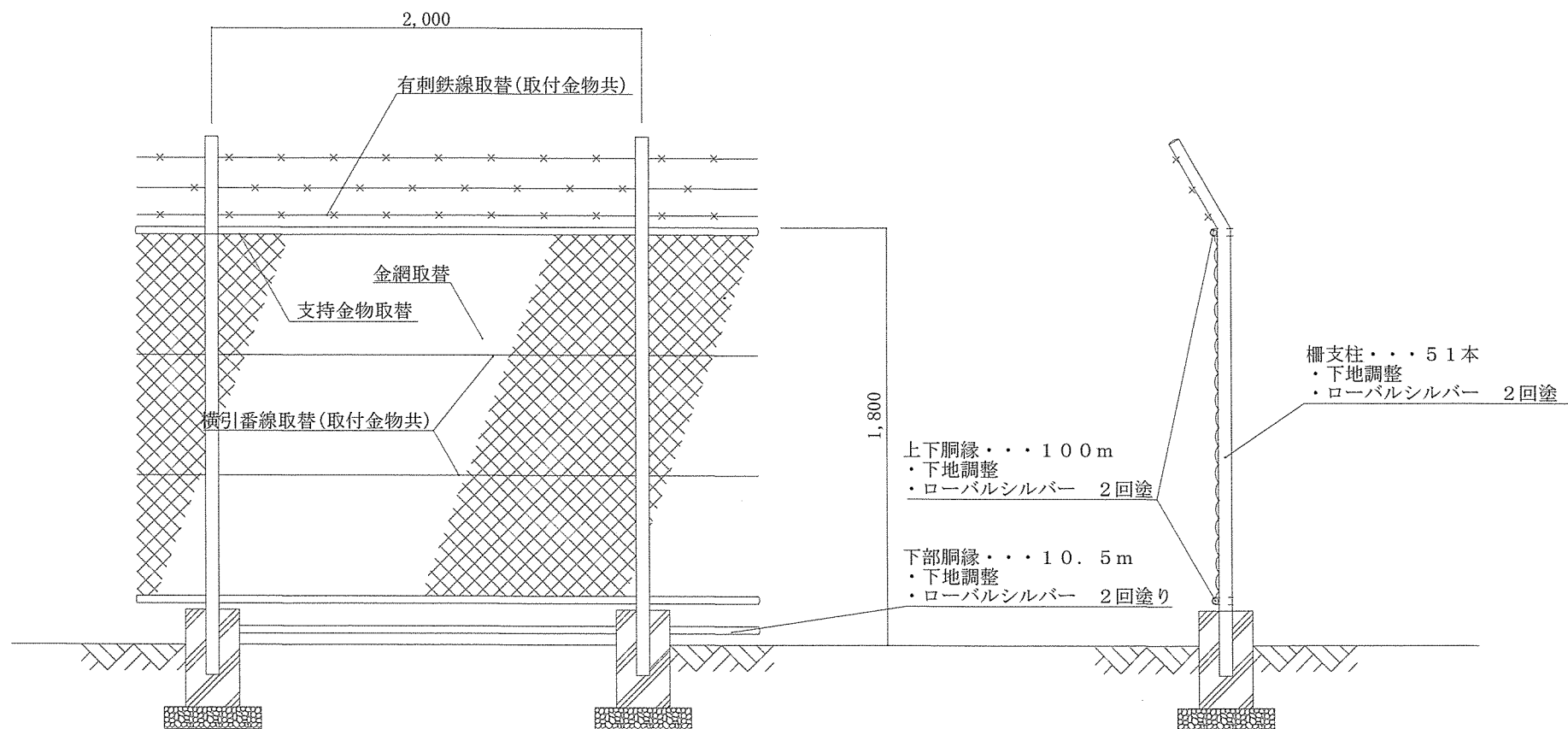
内柵詳細図 1 / 30
