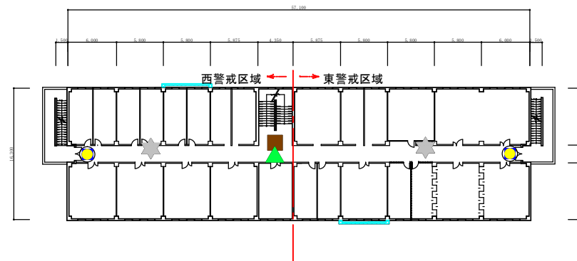
116号A号隊舎 4階平面図
