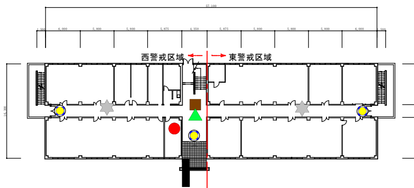
116号A号隊舎 1階平面図
