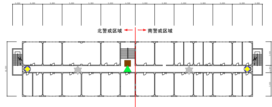
129号D号隊舎 3階平面図
