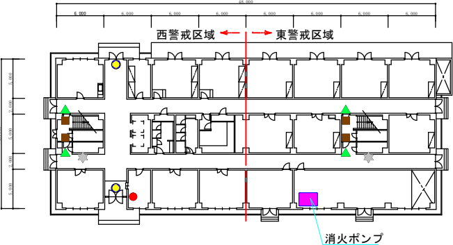
137号E号隊舎 1階平面図
