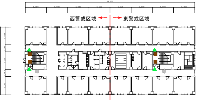
137号E号隊舎 3階平面図
