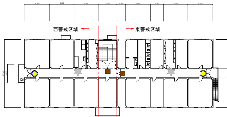
107号WAC隊舎 2 階平面図
