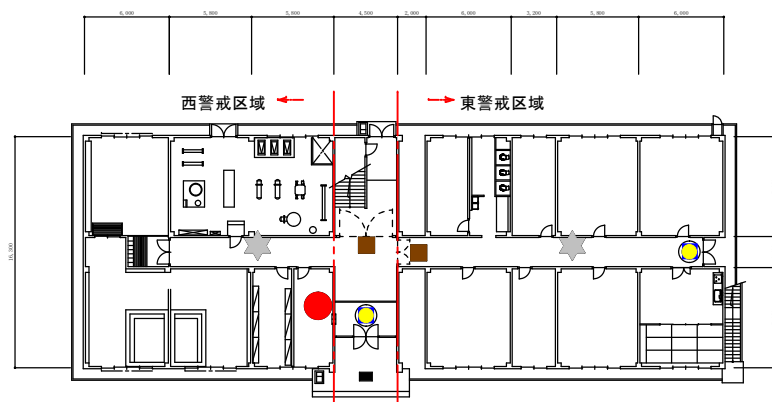
107号WAC隊舎 1 階平面図
