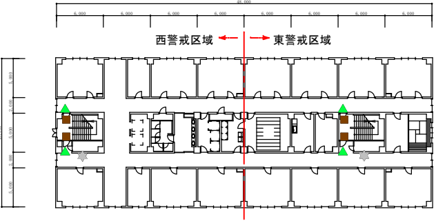
137号E号隊舎 4階平面図
