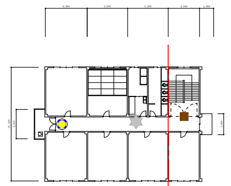
107号WAC隊舎 4 階平面図
