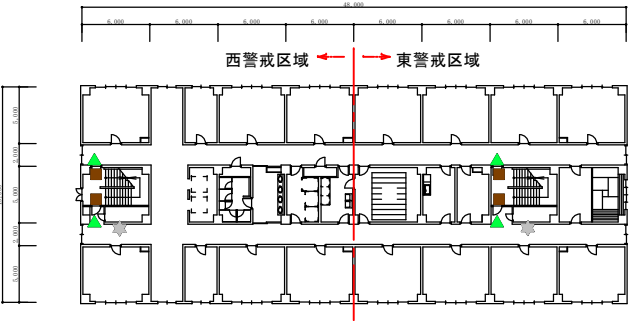
137号E号隊舎 6階平面図
