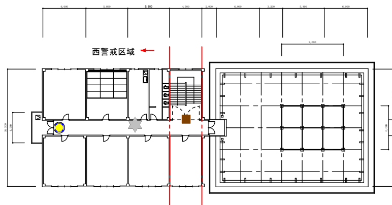
107号WAC隊舎 3 階平面図
