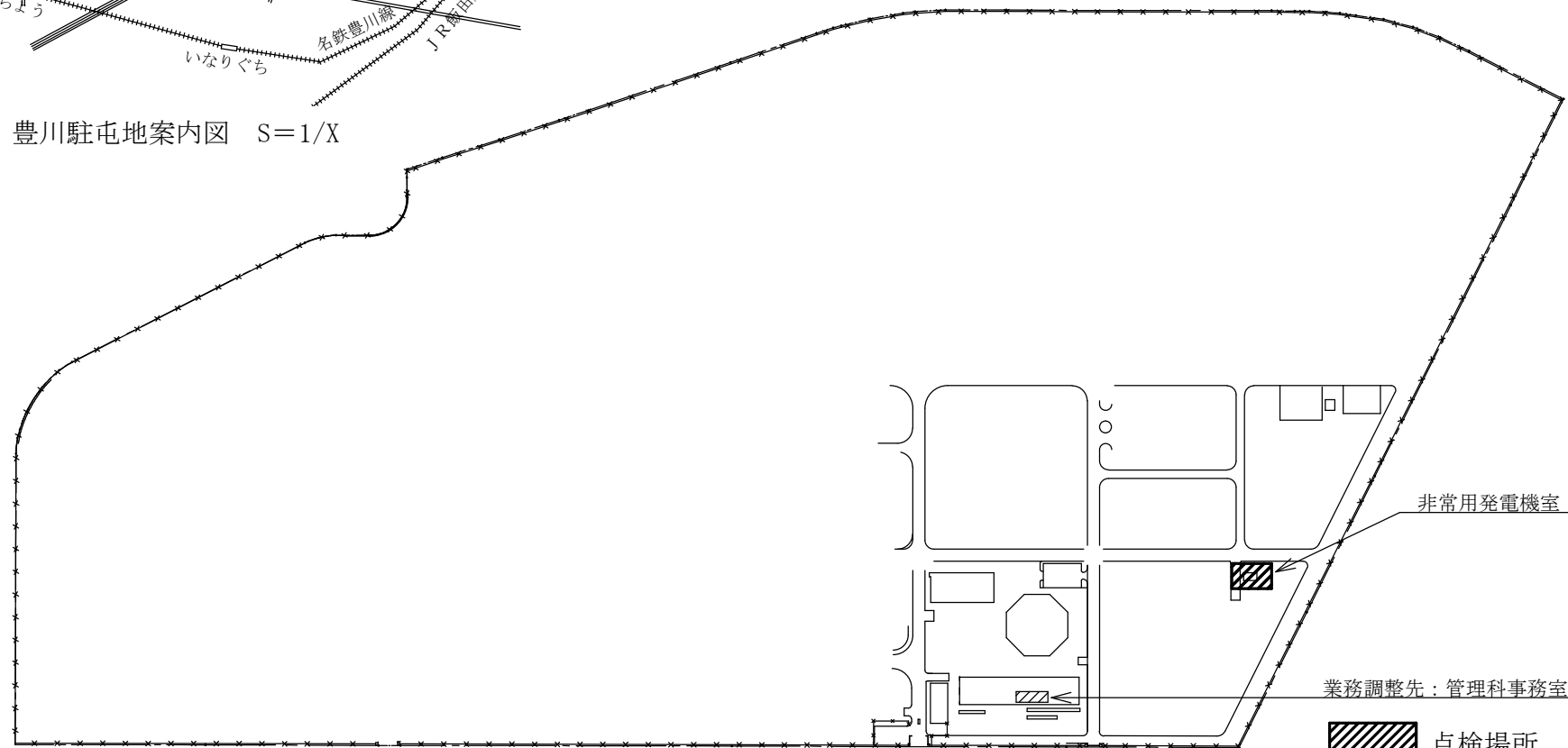
豊川駐屯地配置図 S=1/4500
