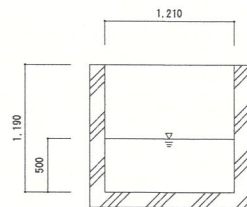
No.1 断面図 (既設洗車場)
