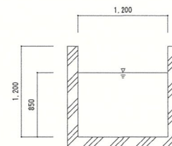
No.2 断面図 (土砂分離槽)
