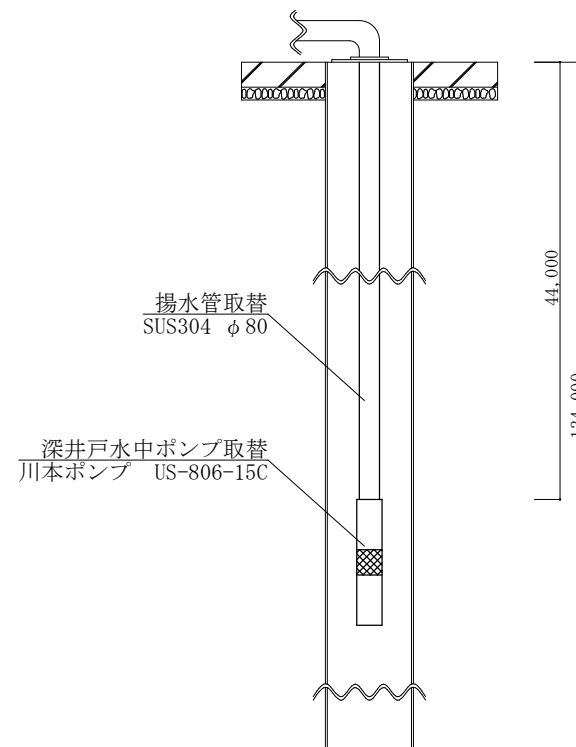
井戸内配管詳細図 S=1：20
