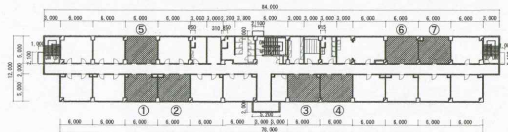
117号隊舎2F平面図 S=1/500
