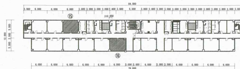
117号隊舎5F平面図 S=1/500
