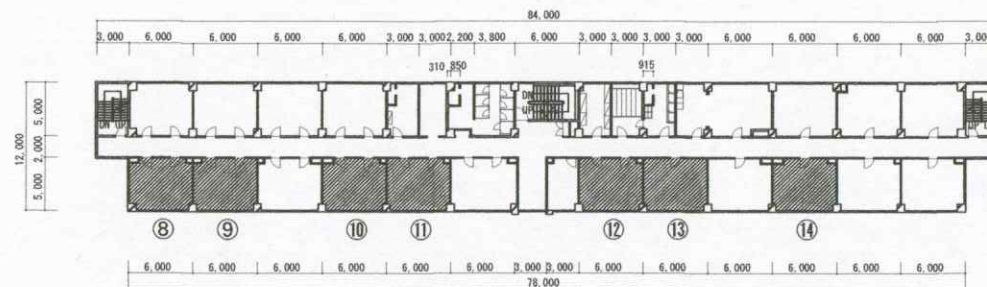
117号隊舎3F平面図 S=1/500
